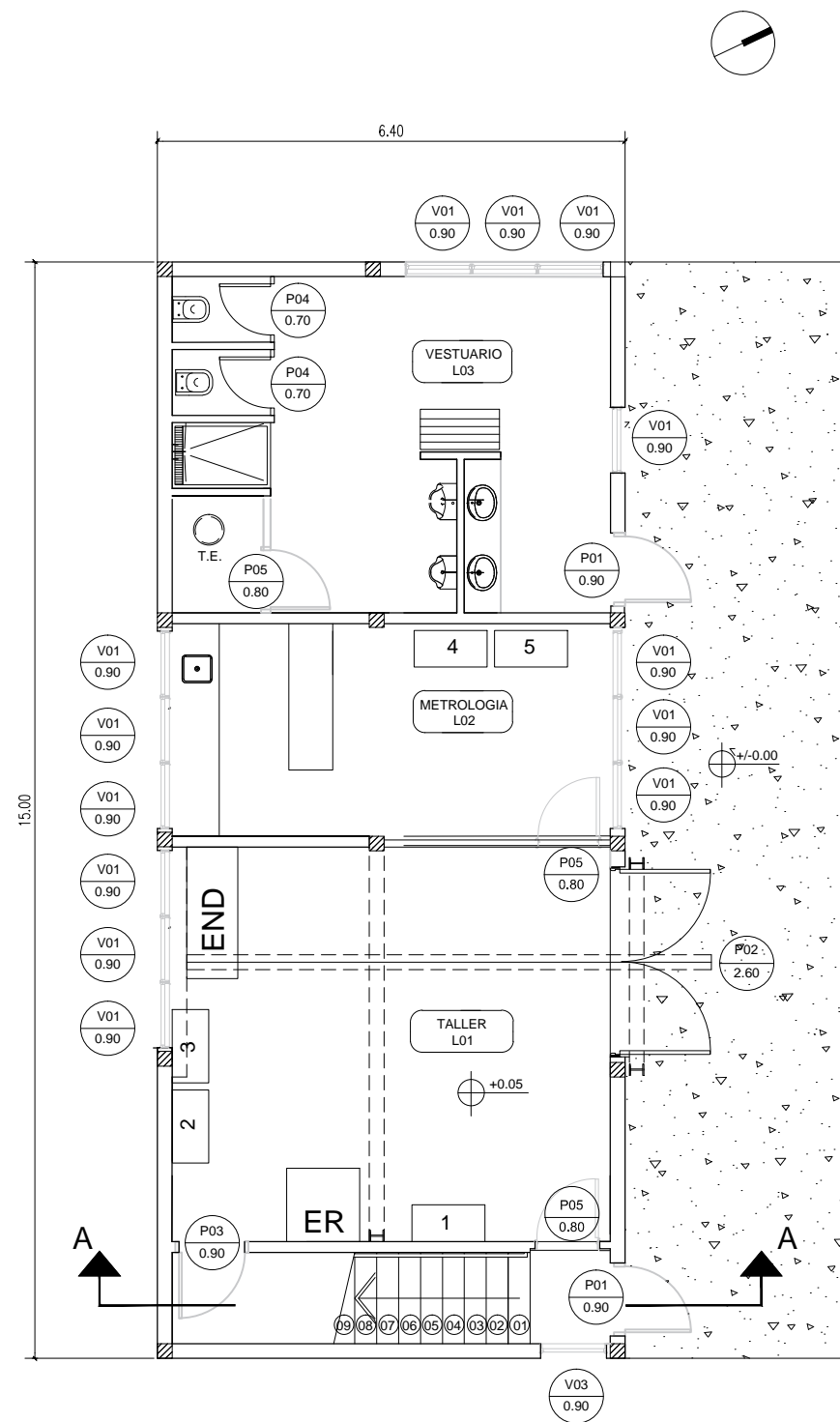
PLANTA BAJA
