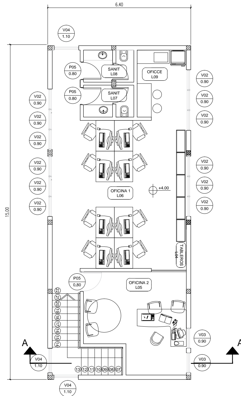
PLANTA ALTA
