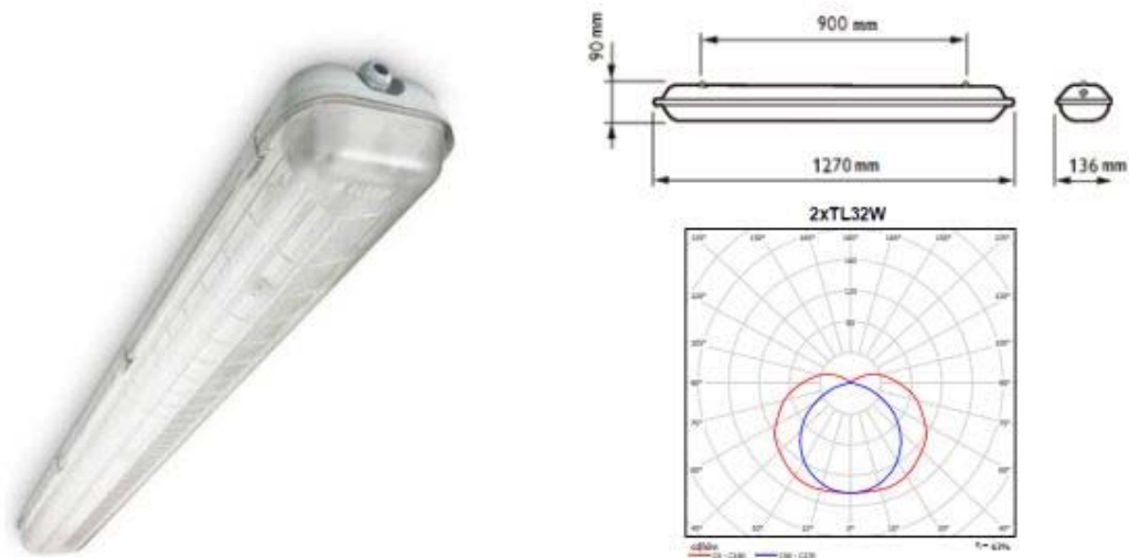
Imagen 10 - Luminaria de referencia
