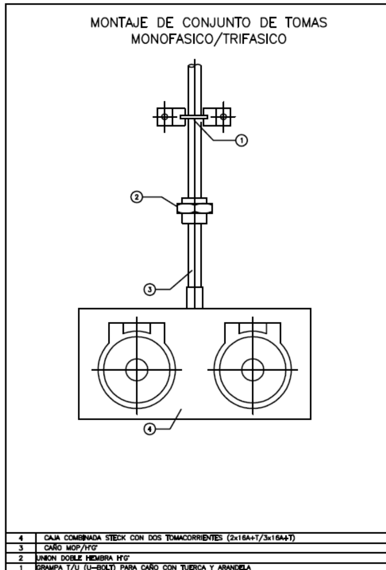
Imagen 12 - Ilustración de referencia: Montaje de tomas
