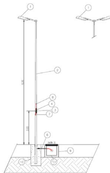
Imagen 8 – Detalle columna de Iluminación (Ver Anexo X)
