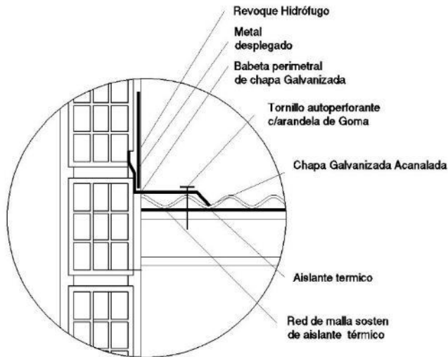
Imagen 10 – Babetas perimetrales
