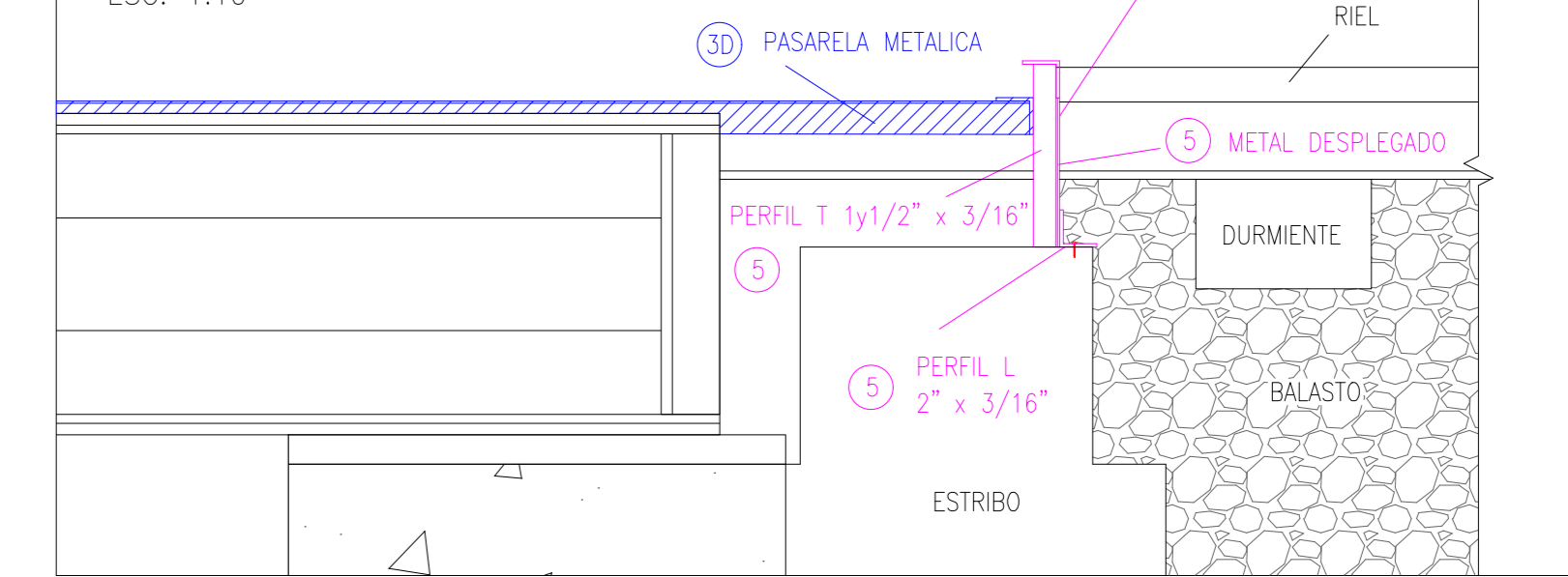
DETALLE 2 - GUARDABALASTO - CORTE ESC: 1:10
