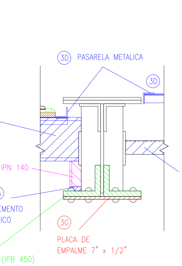
CORTE B-B ESC: 1:10
