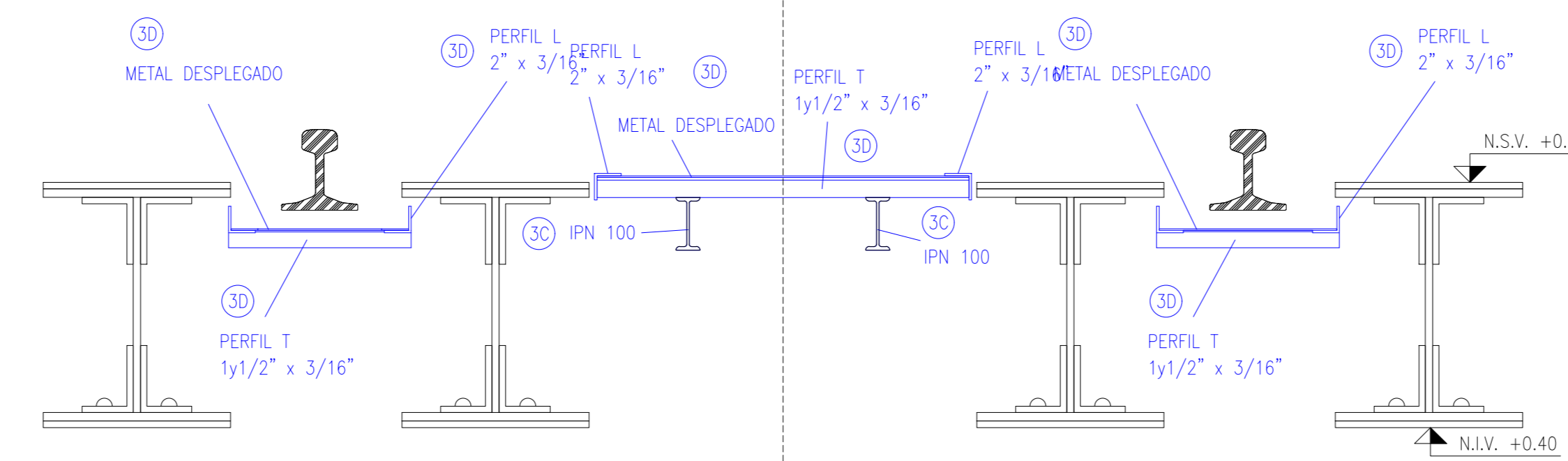
CORTE B-B ESC: 1:10
