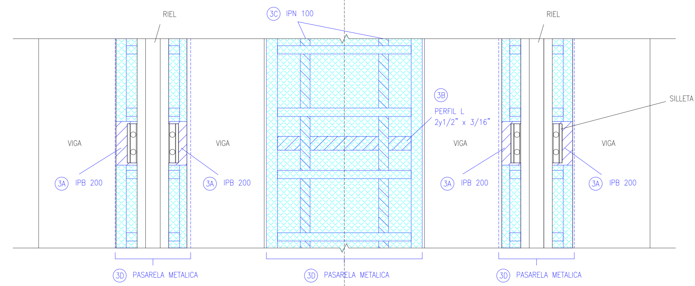
PLANTA ESC: 1:10
