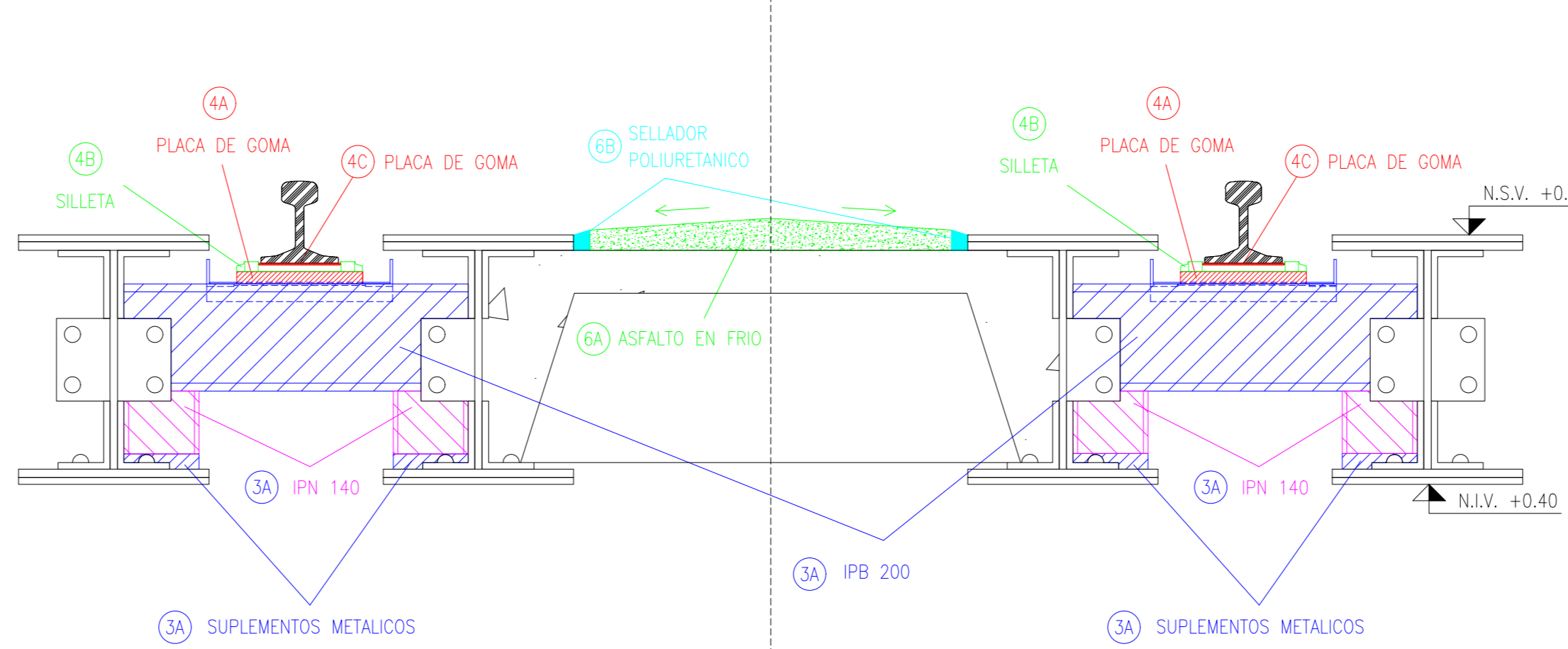
CORTE B-B ESC: 1:10
