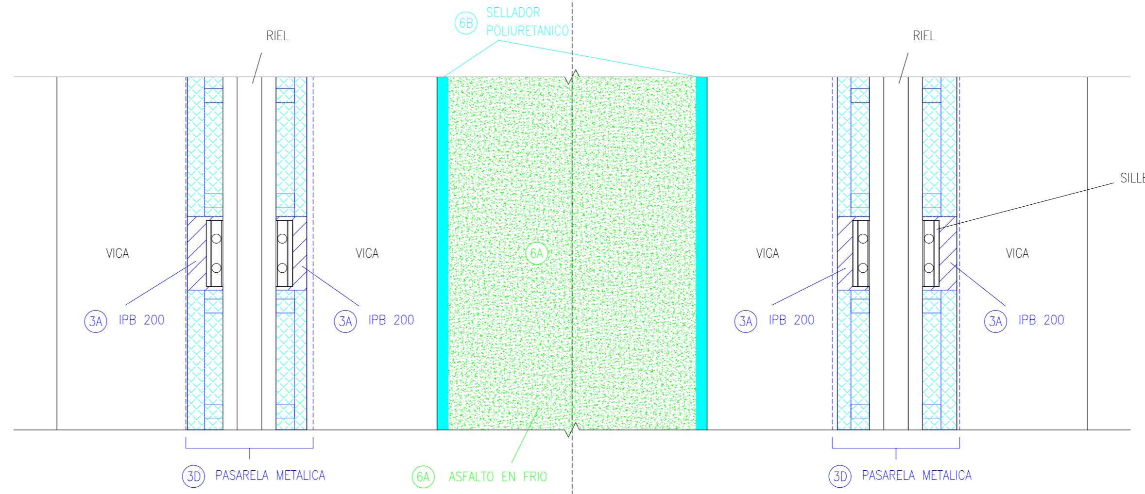
PLANTA ESC: 1:10
