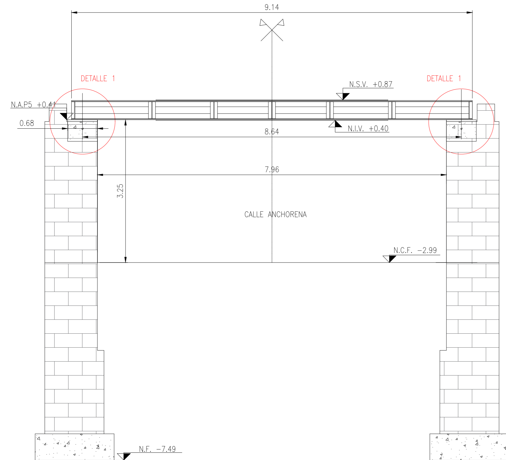
VISTA 1-1 ESC: 1:50
