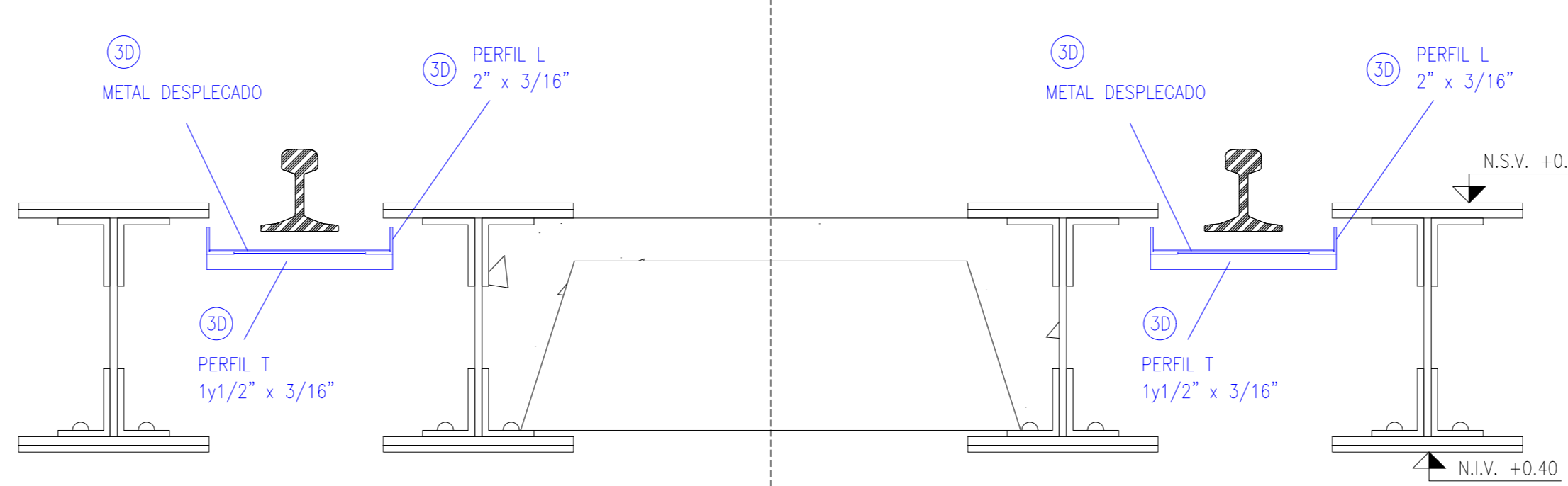
CORTE B-B ESC: 1:10
