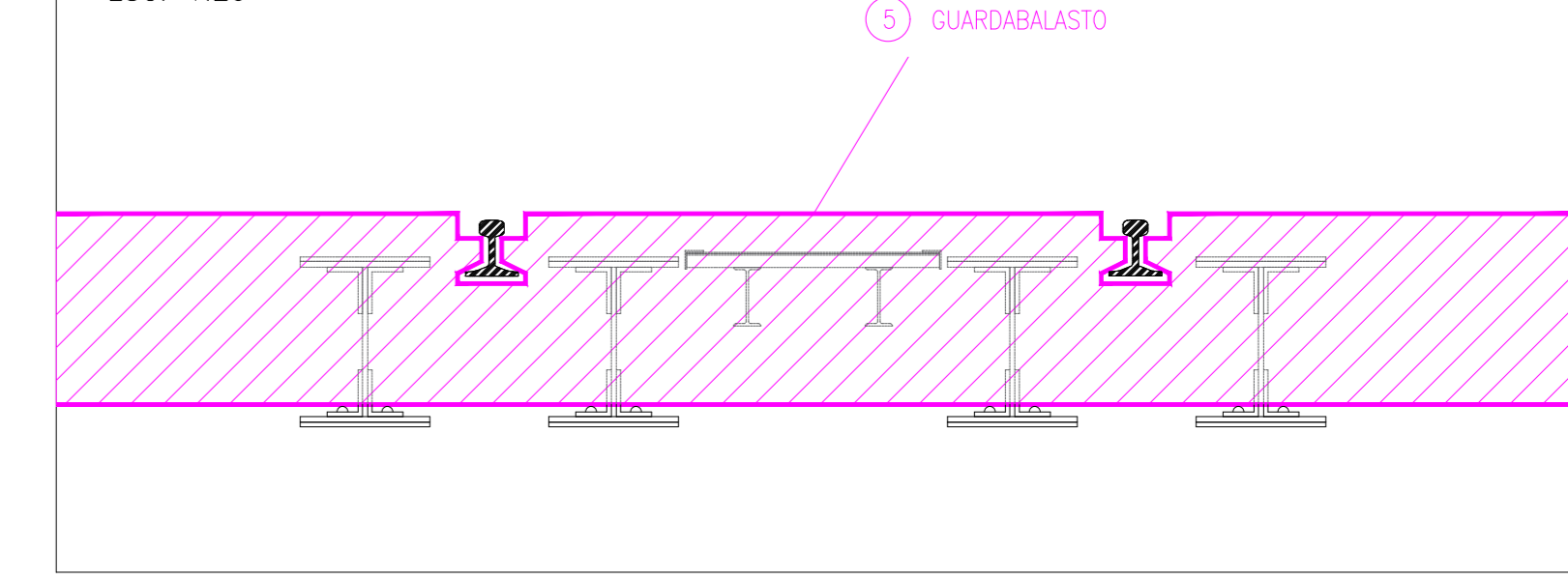
DETALLE 2 - GUARDABALASTO - VISTA ESC: 1:20
