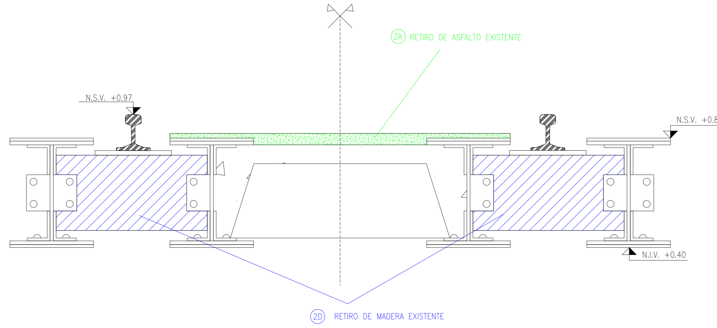
CORTE A-A ESC: 1:10
