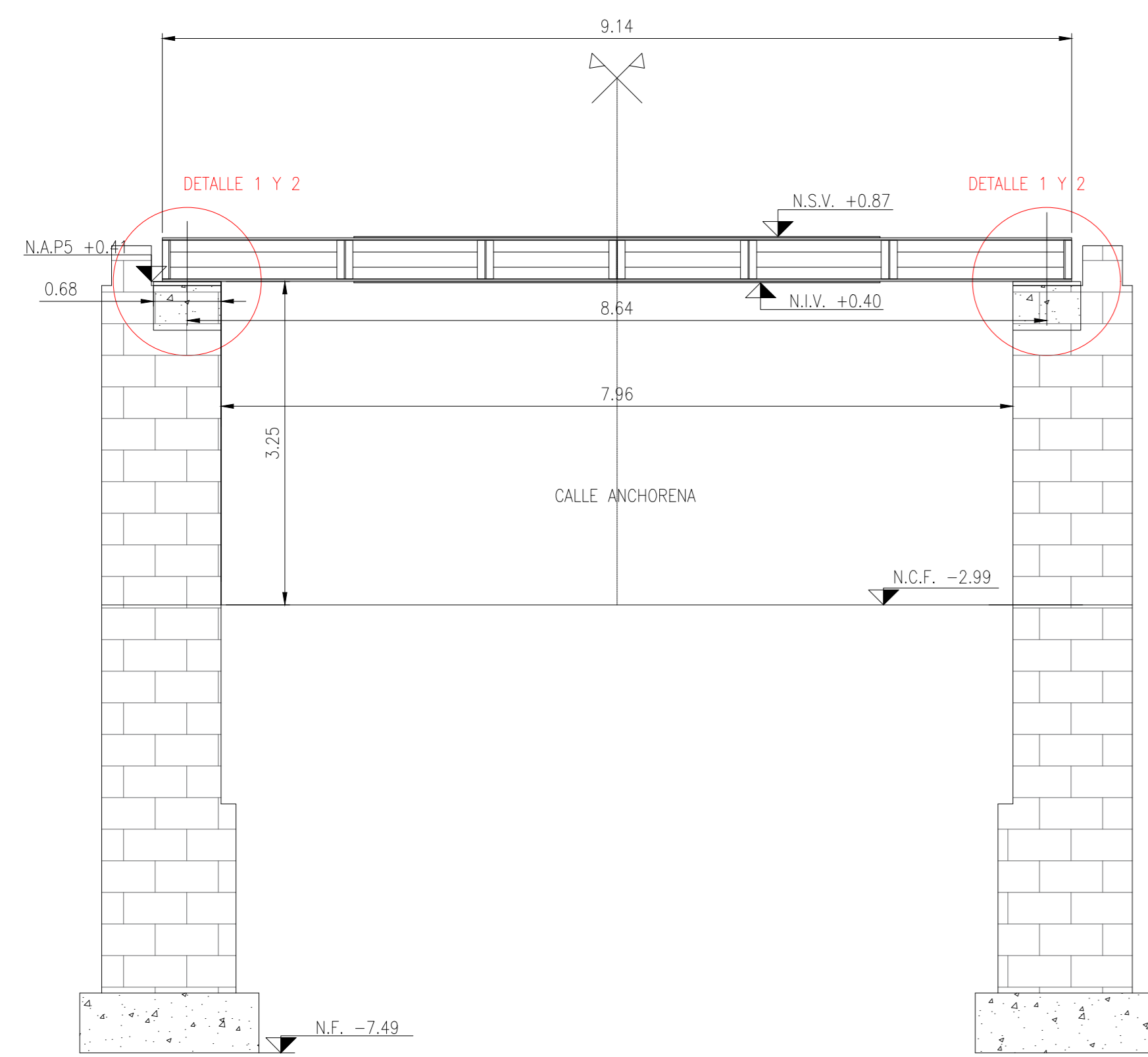
VISTA 1-1 ESC: 1:50
