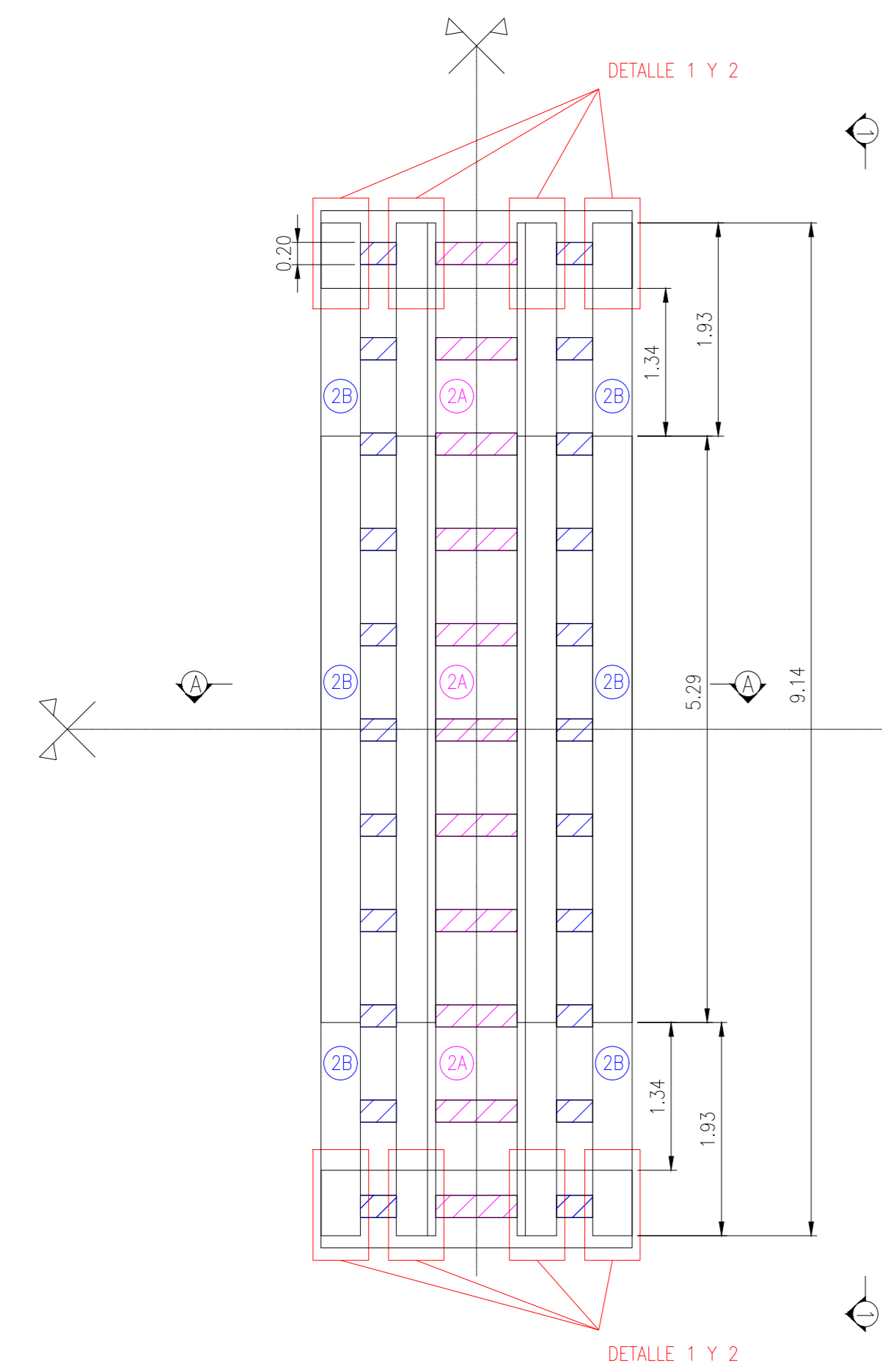
PLANTA GENERAL +0.41 ESC: 1:50
