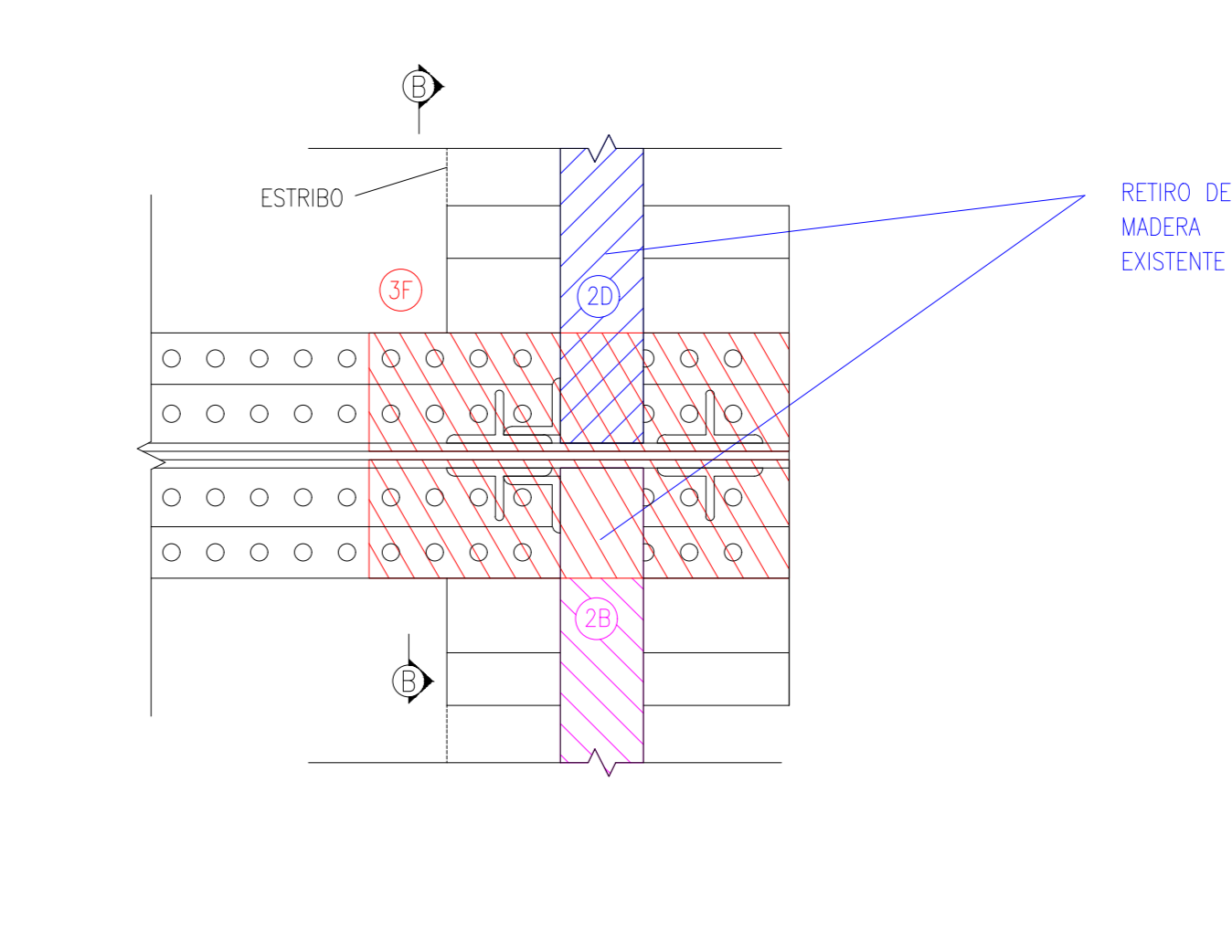
PLANTA APOYO +0.60 - DETALLE 1 ESC: 1:10
