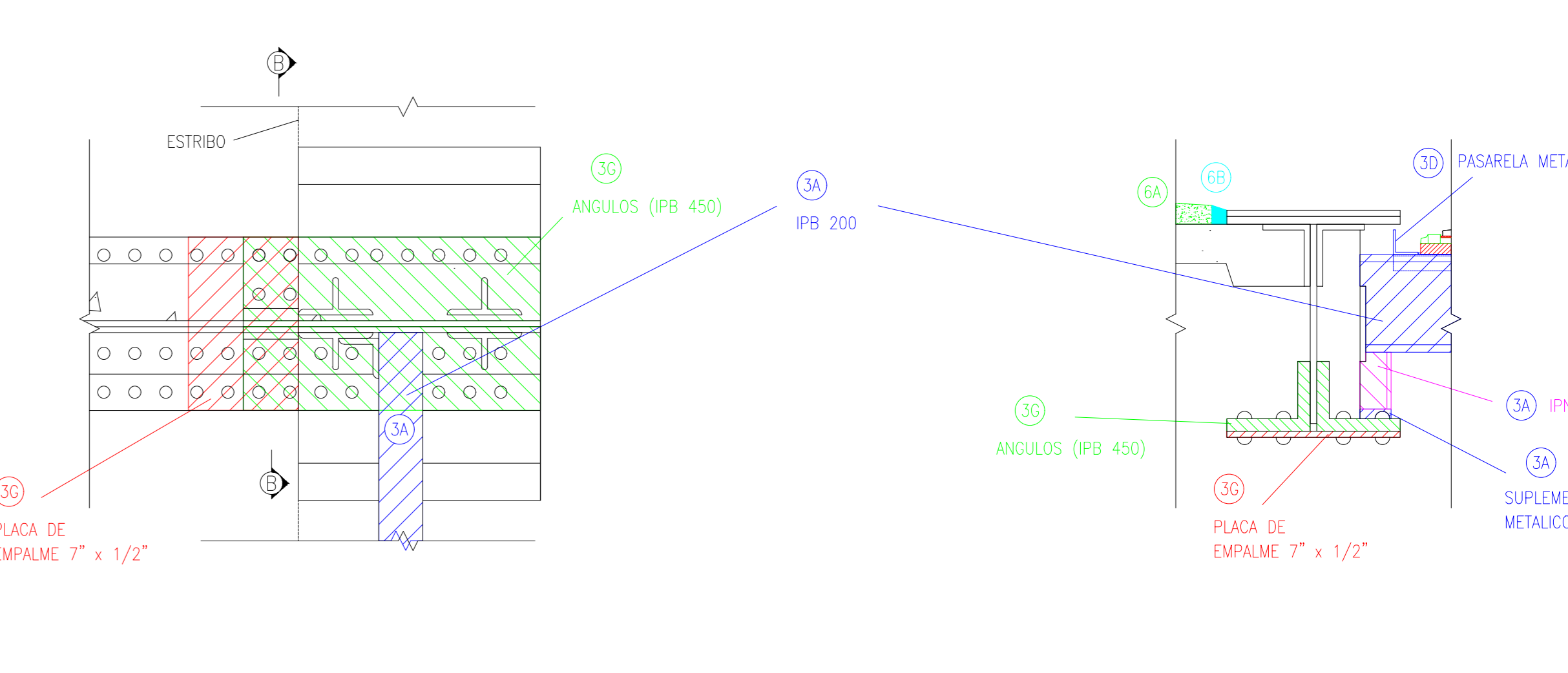
PLANTA APOYO +0.60 - DETALLE 1 ESC: 1:10
