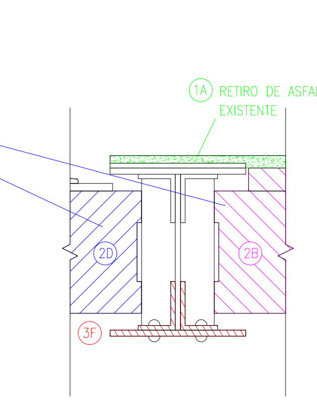
CORTE B-B ESC: 1:10
