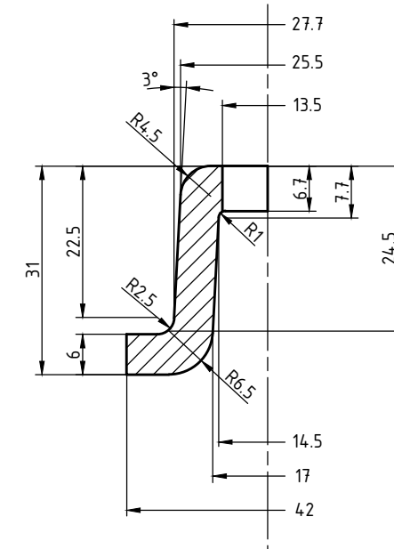
SECCIÓN A-B ESCALA 1:1
