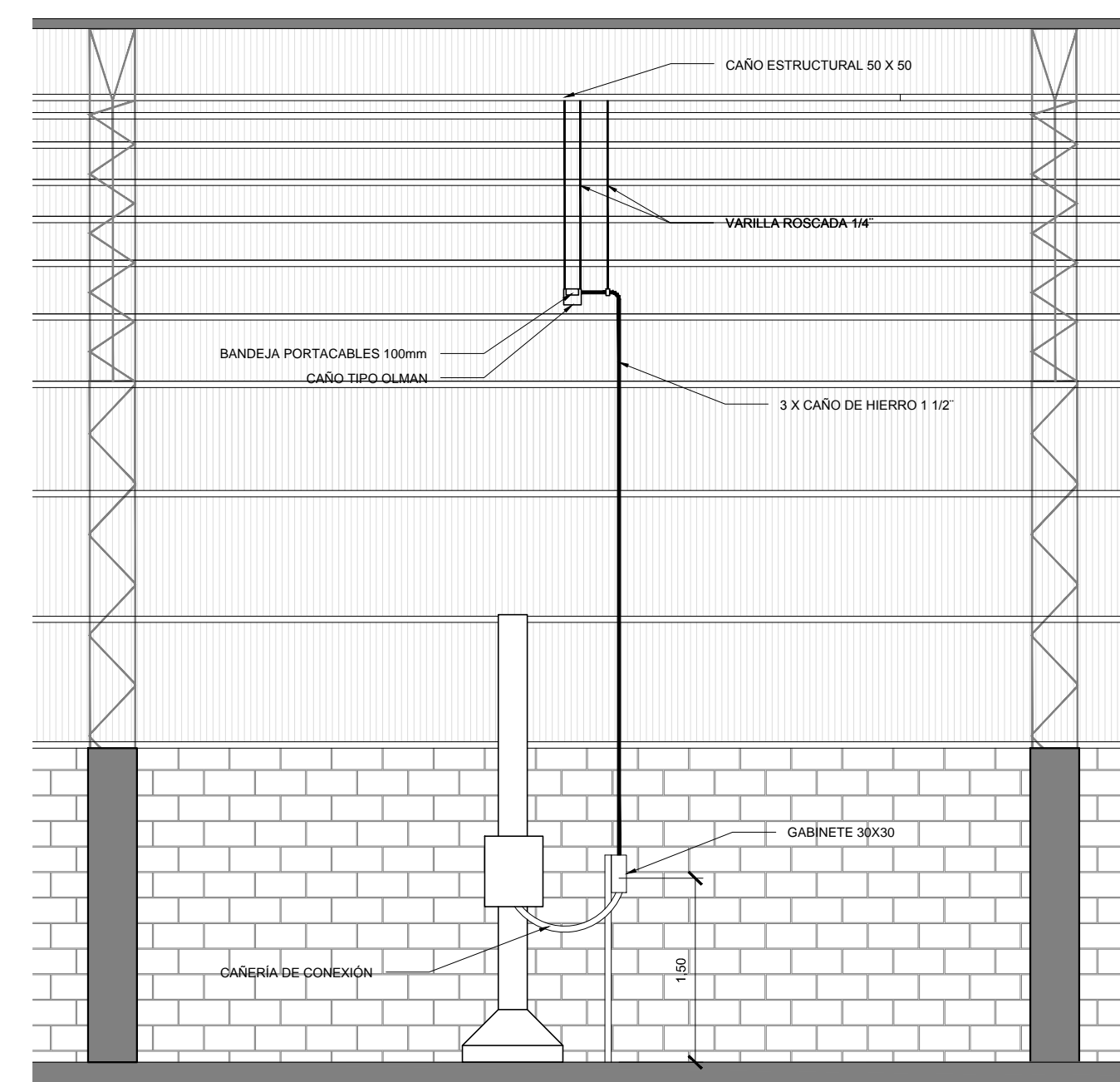
DETALLE DE CAÑERIAS DE BAJADA A GATO ELECTROMECANICO ESC. 1/50
