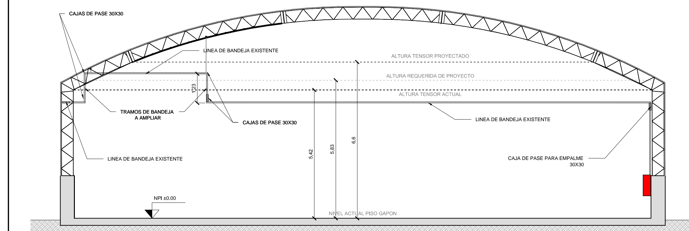
CORTE PERPENDICULAR - TRAMO A ELEVAR BANDEJA EXISTENTE ESC. 1/100
