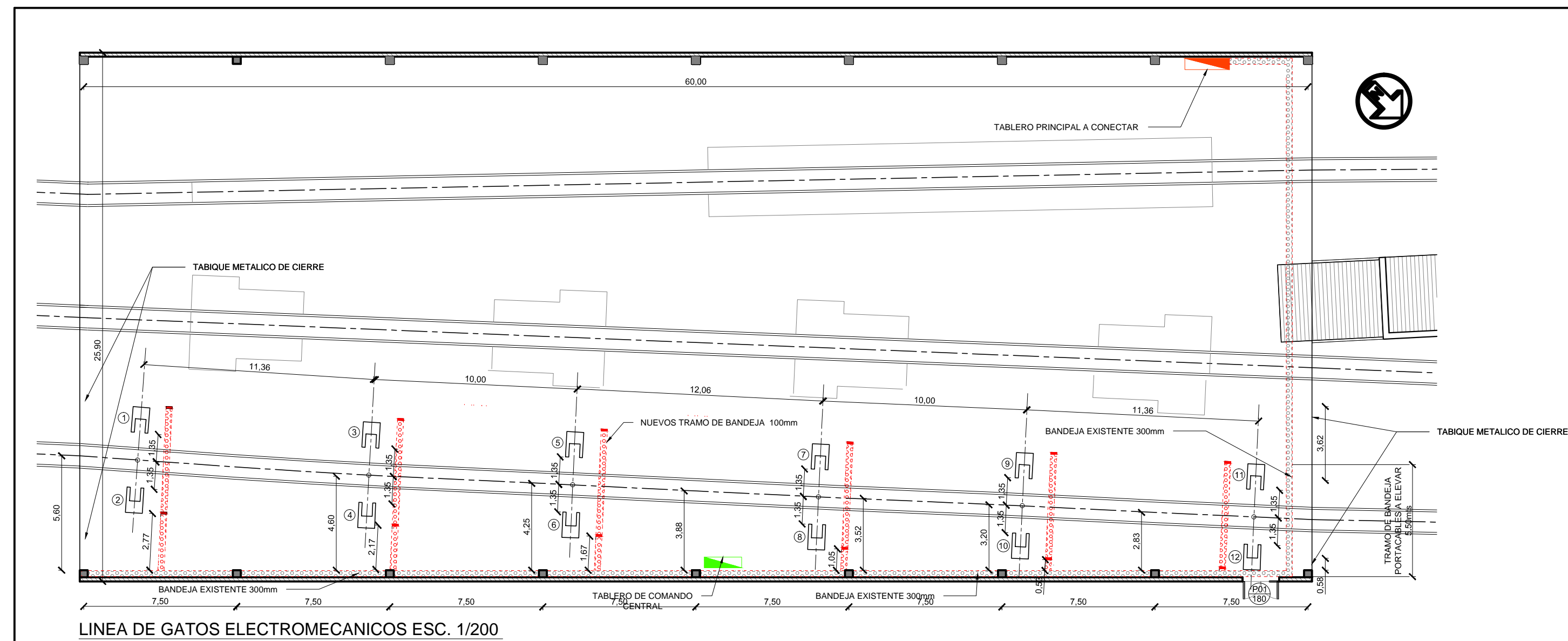
LINEA DE GATOS ELECTROMECANICOS ESC. 1/200
