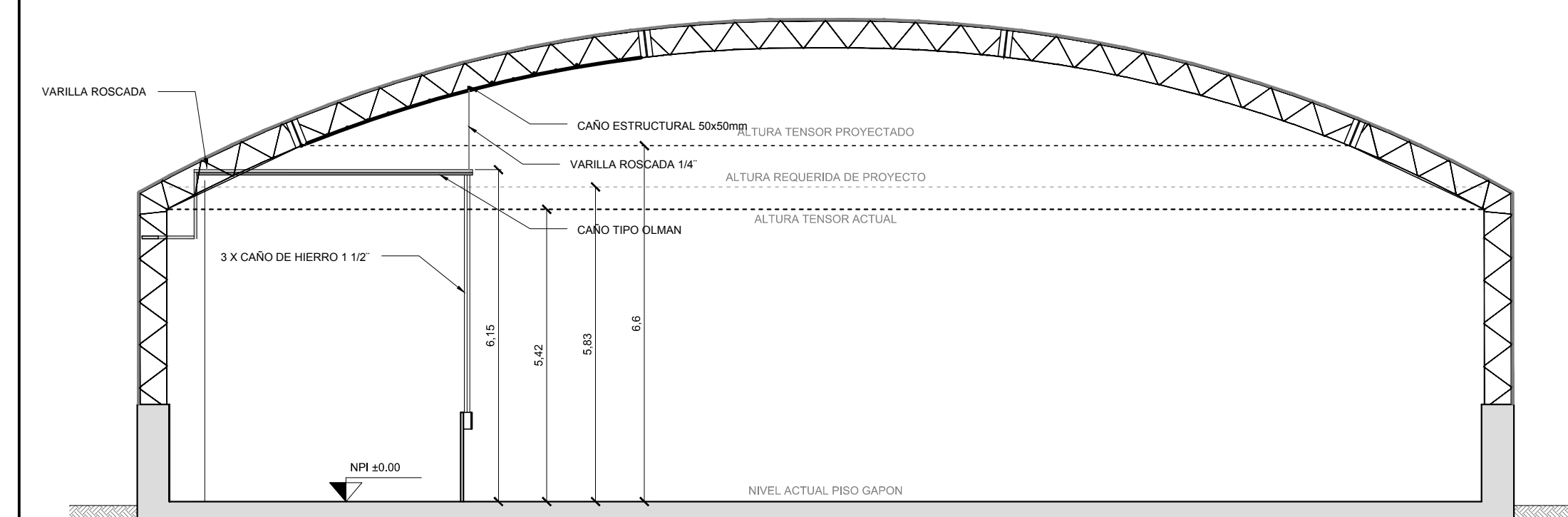
CORTE PERPENDICULAR - PORTICO DE BANDEJA PORTACABLE ESC. 1/100
