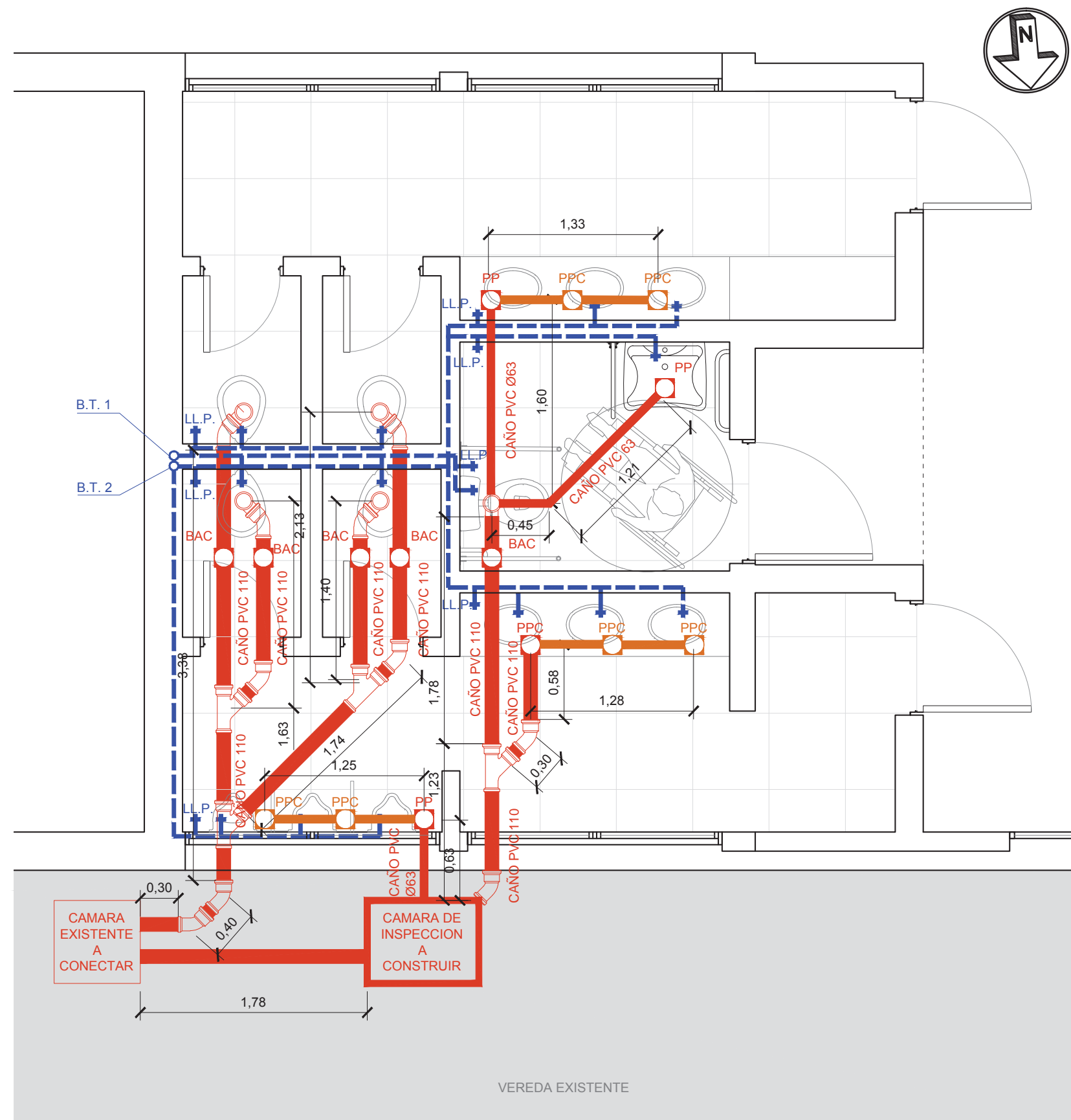
ANTEPROYECTO INSTALACION SANITARIA ESC. 1/50
