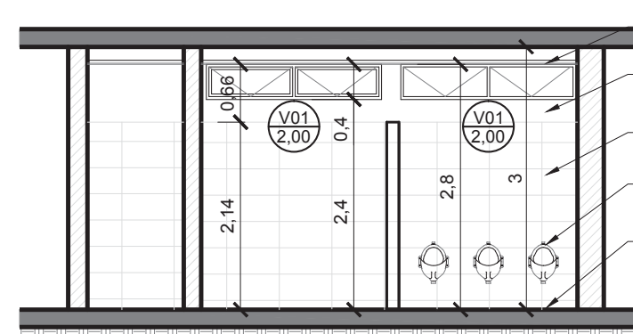
ANTEPROYECTO CORTE A-A ESC. 1/100
