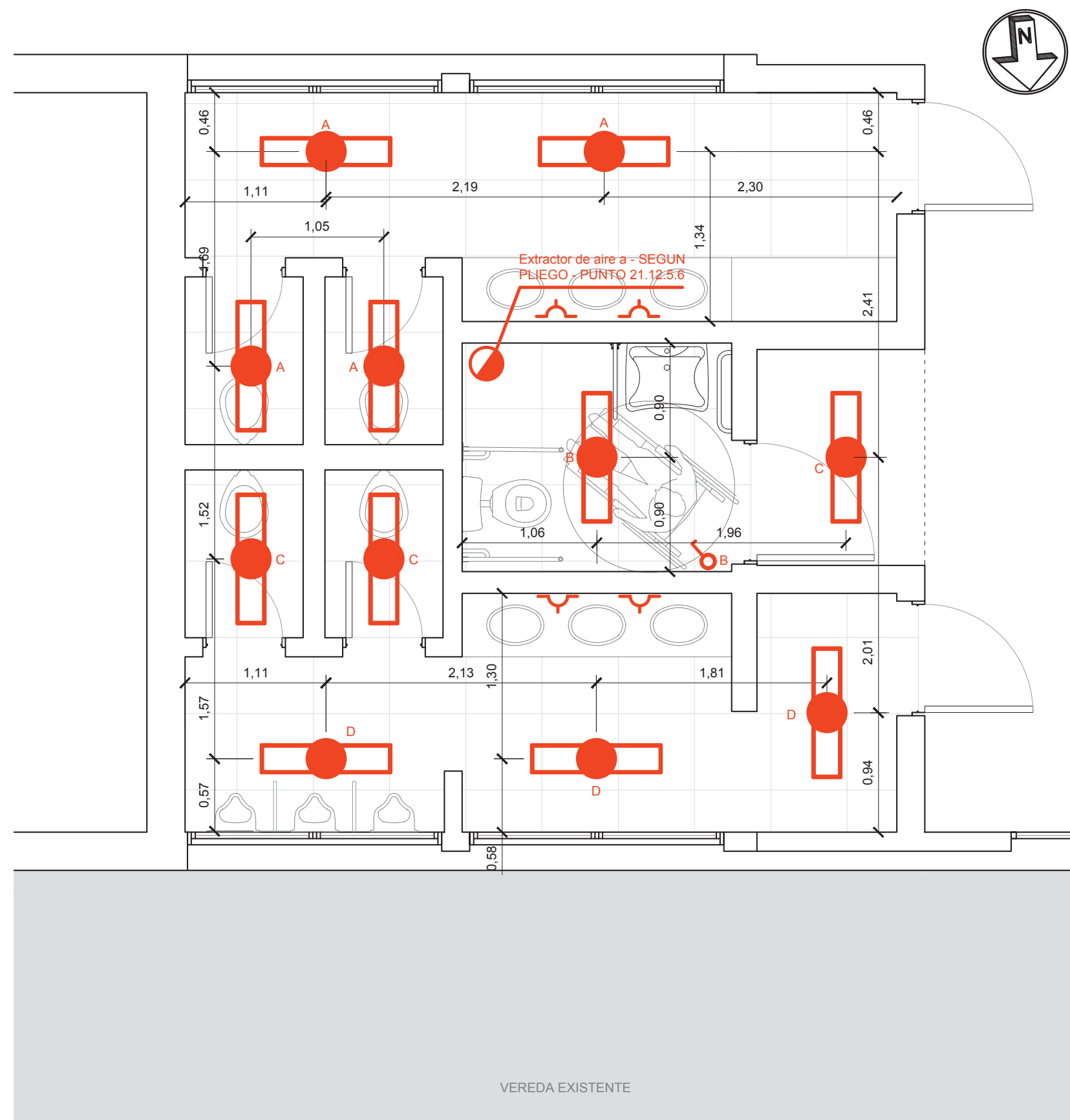
ANTEPROYECTO INSTALACION ELECTRICA ESC. 1/50
