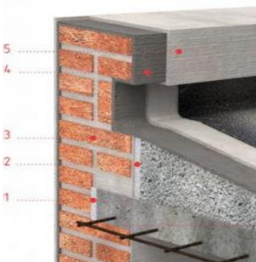
Imagen ilustrativa: Detalle de muro de carga, (1-Losa, 2-Contrapiso, 3-carga, 4-aislacion hidrófuga y 5-revoques).
