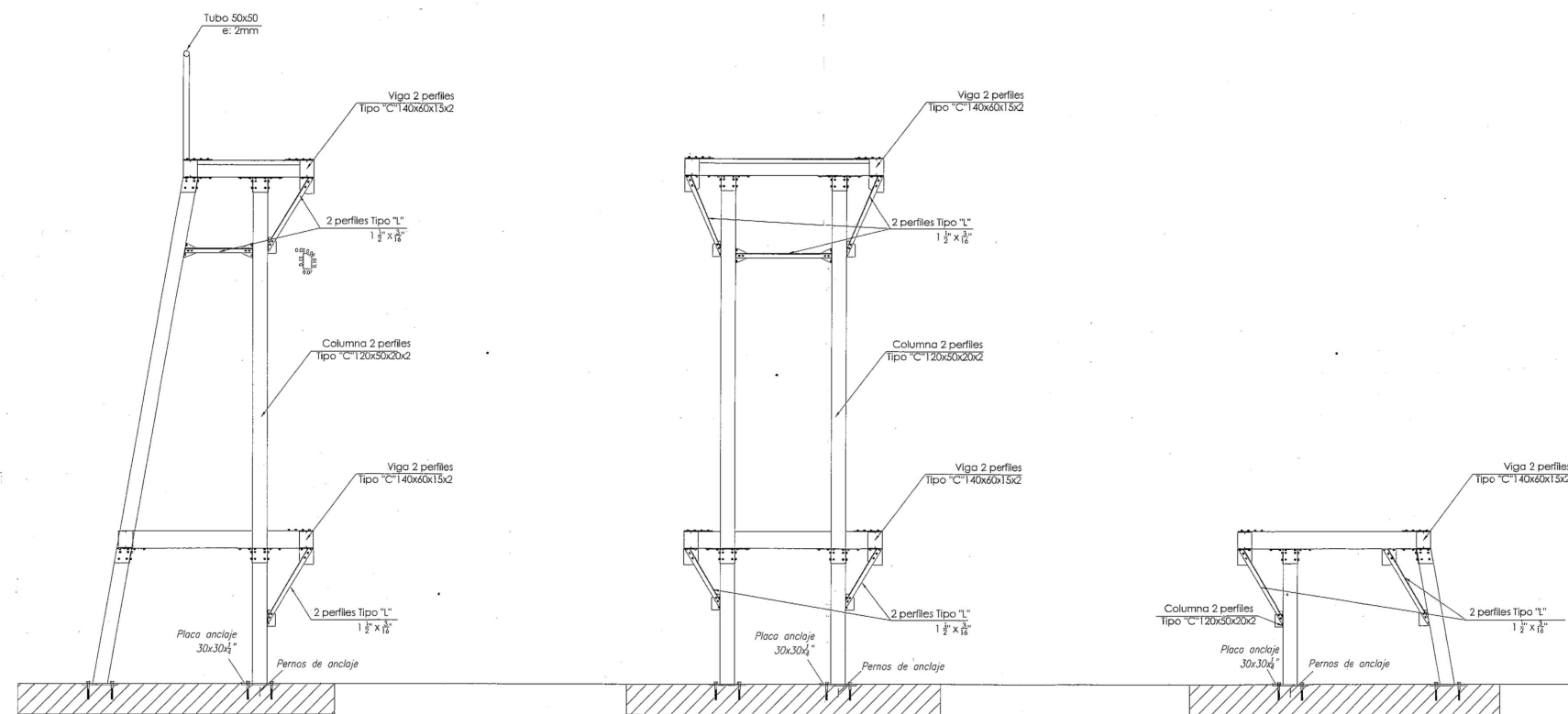
PASARELA EXTREMA IZQ. ESC. 1 : 25
