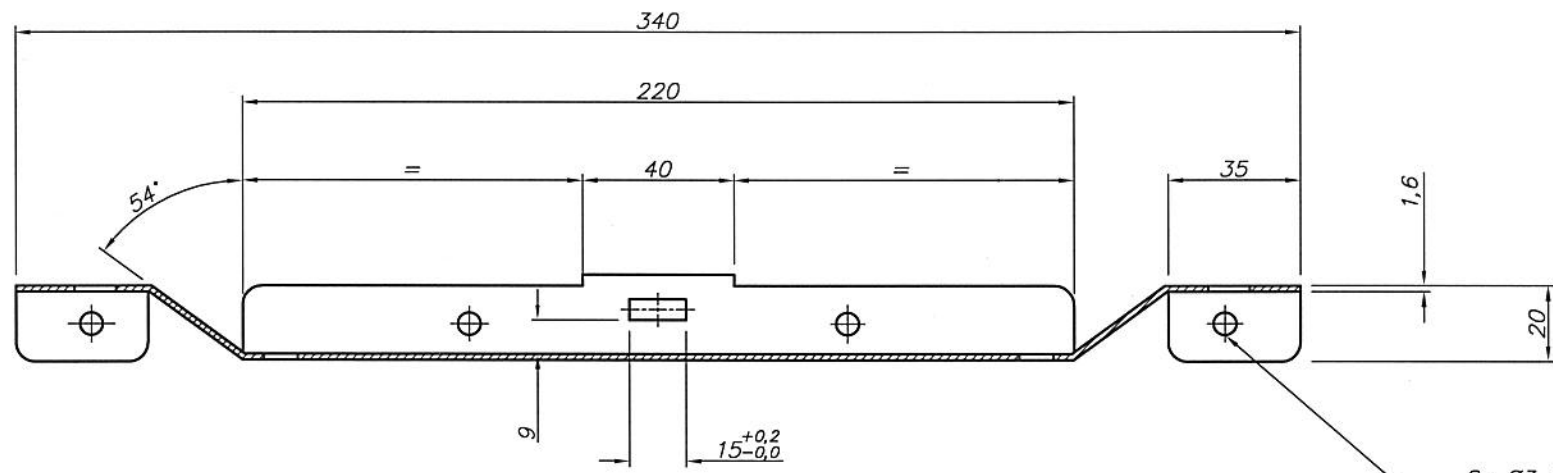
CORTE A-A
