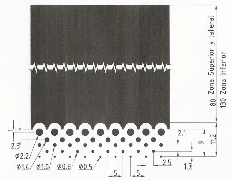
Detalle de serigrafía perimetral (Diseño opcional)
