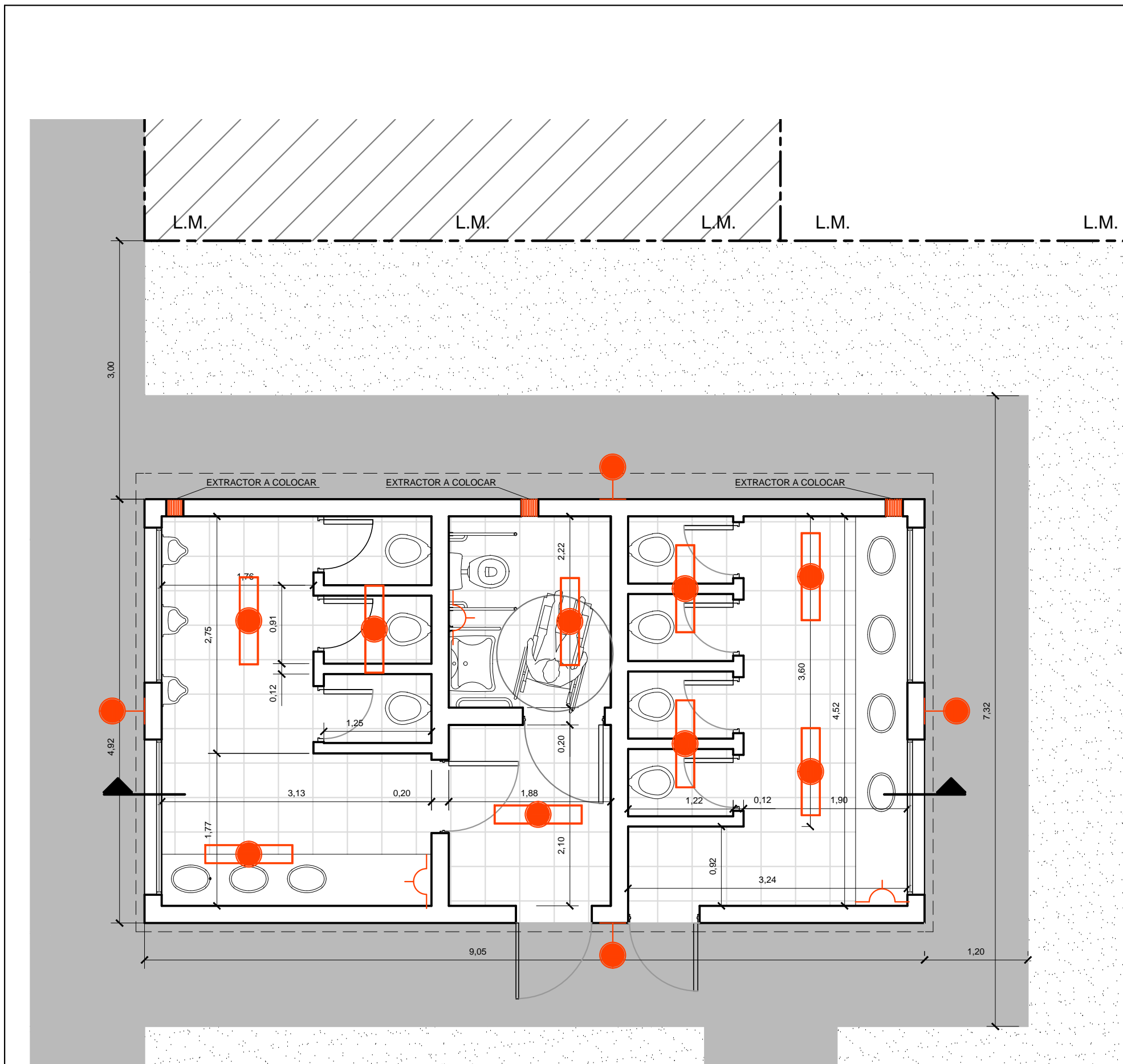
INSTALACION ELE CTRICA - PLANTA BAJA 1:100
