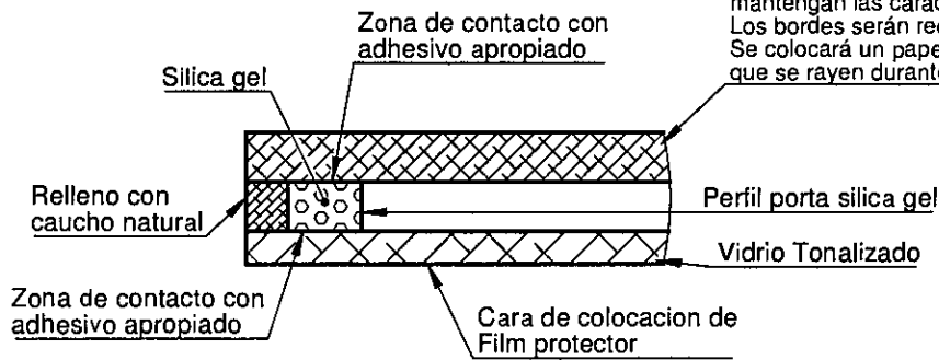
DETALLE A
