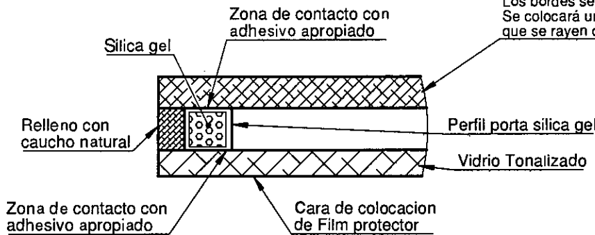
DETALLE A
