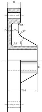
CORTE A-A
