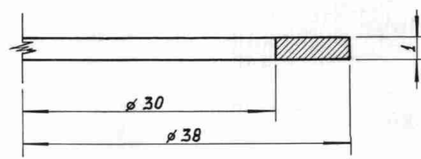
DETALLE DE LA PIEZA Nº 5 Esc. 5:1-
