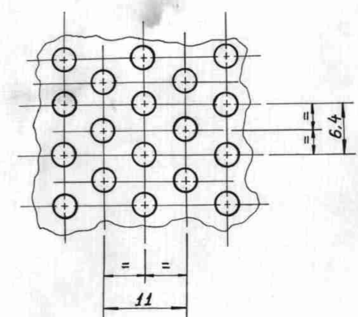
DETALLE DEL PERFORADO DE LA PIEZA Nº 9
