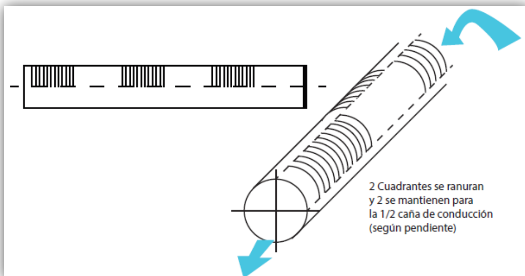
Fig. 1 Esquema de Ranuras.
