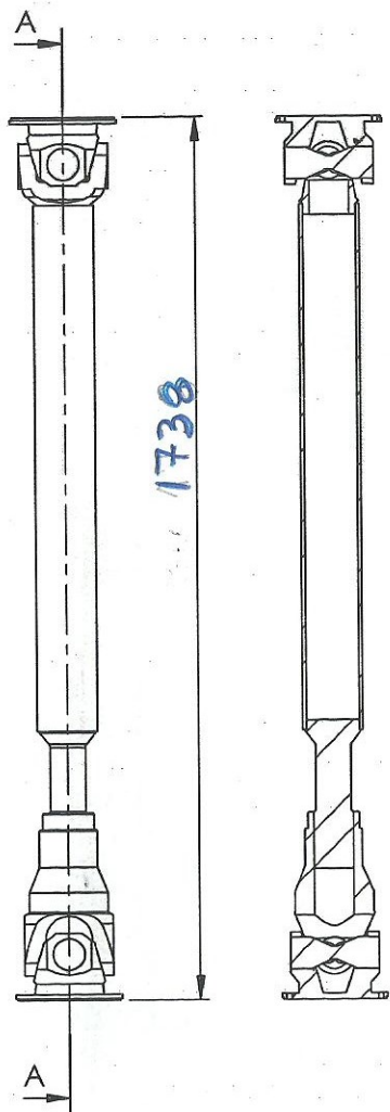
SECCIÓN A-A ESCALA 1 : 15
