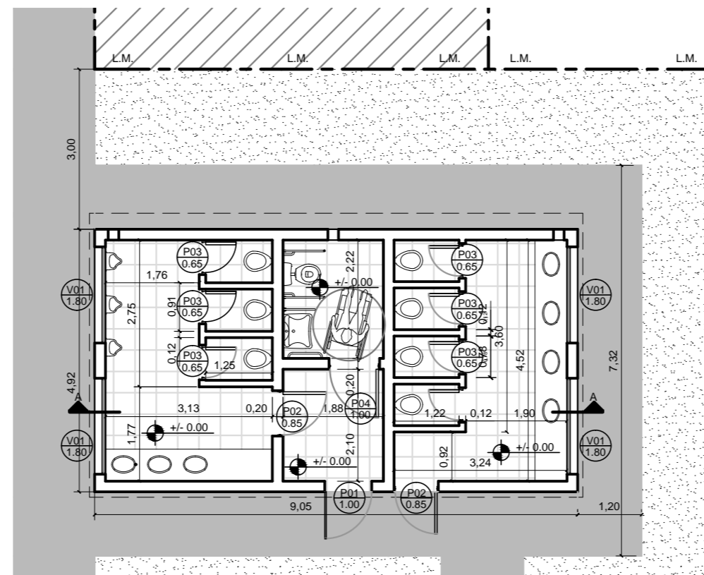
ANTEPROYECTO - PLANTA 1:100
