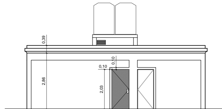
ANTEPROYECTO - VISTA 1 1:100
