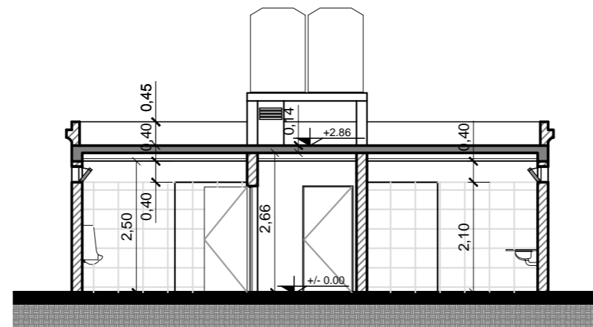
ANTEPROYECTO - CORTE A-A 1:100
