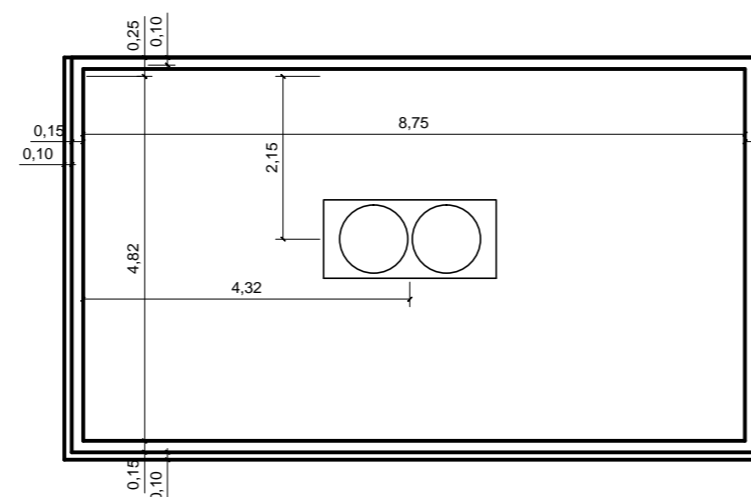
ANTEPROYECTO - PLANTA DE TECHO 1:100
