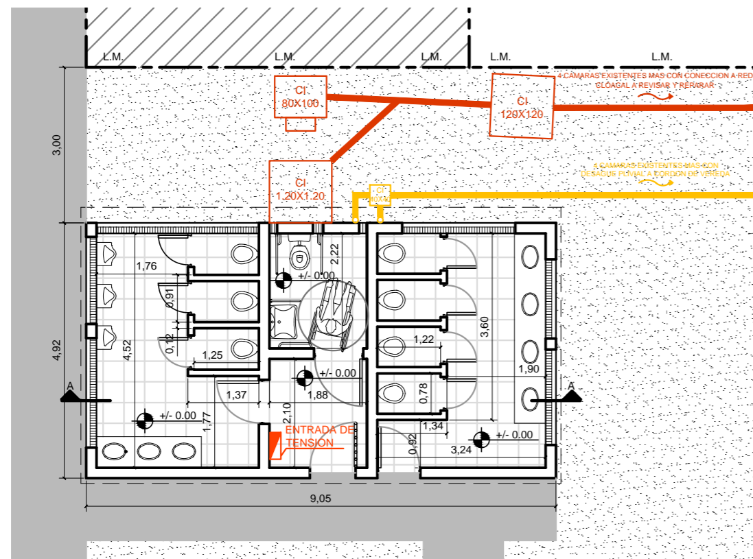
SITUACION ACTUAL - PLANTA 1:100
