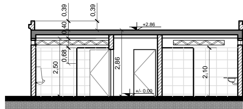
SITUACION ACTUAL - CORTE A-A 1:100
