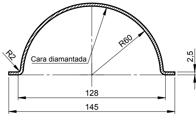
SECCIÓN A-A Escala 1:2
