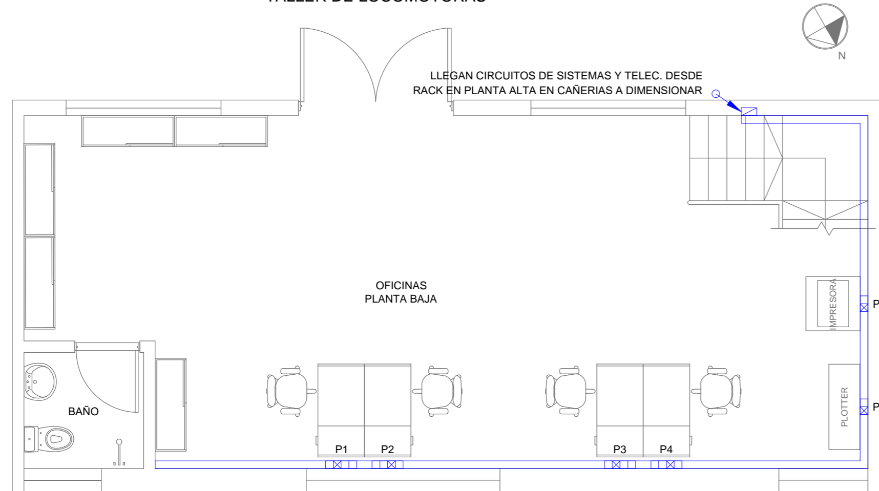
PLANTA BAJA
