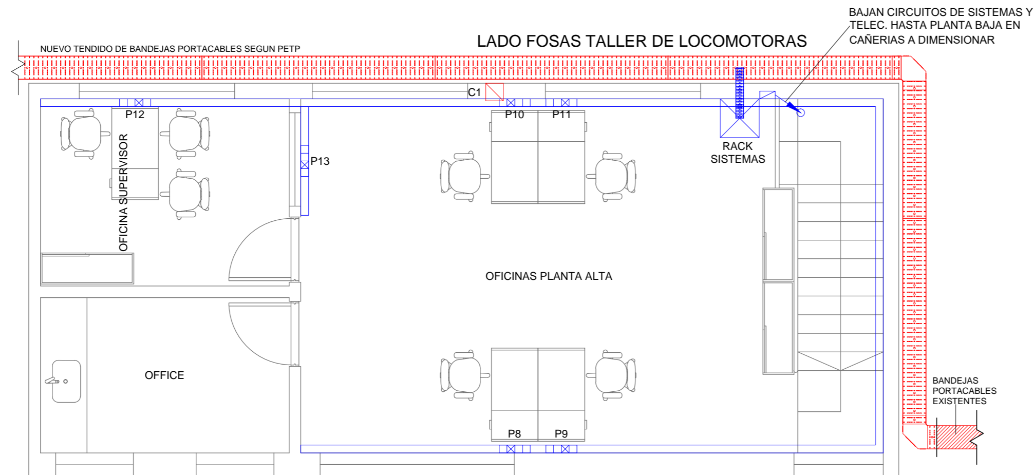
PLANTA ALTA
