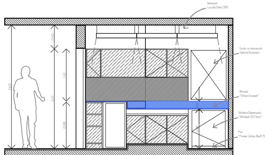
Corte Longitudinal
