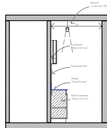
Corte Transversal O2
