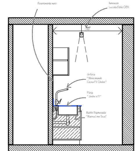
Corte Transversal O3
