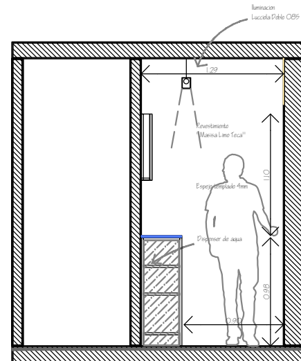
Corte Transversal O1
