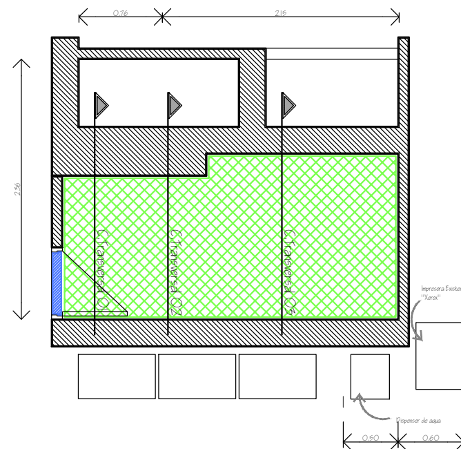
Planta / Solados
