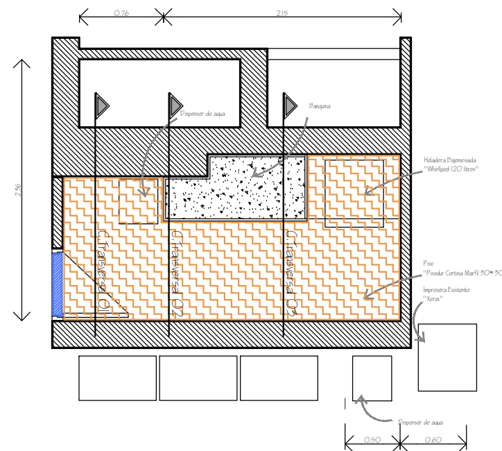
Planta / Solados
