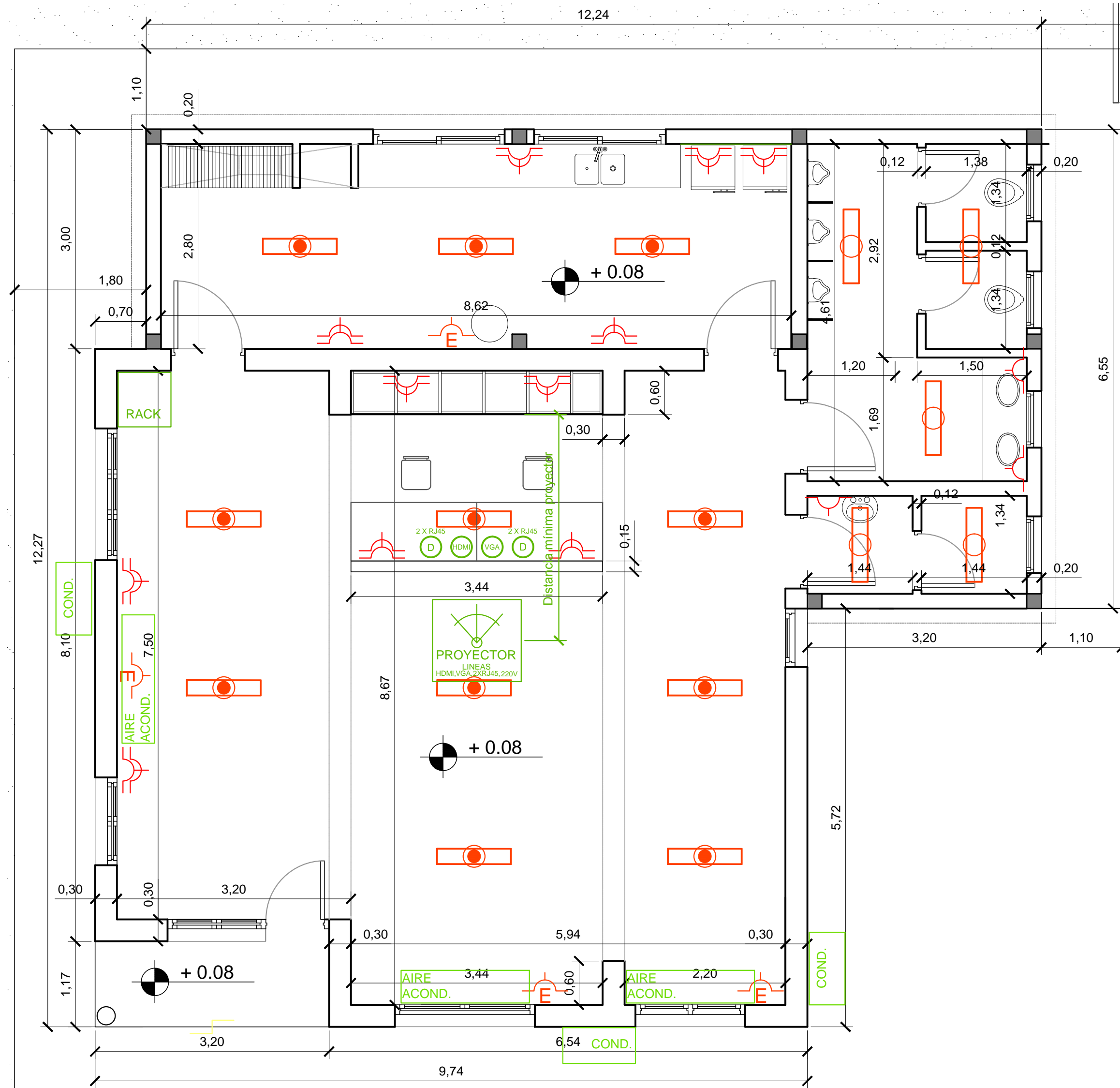
ANTEPROYECTO - INSTALACION ELECTRICA PLANTA BAJA ESCALA 1/50
