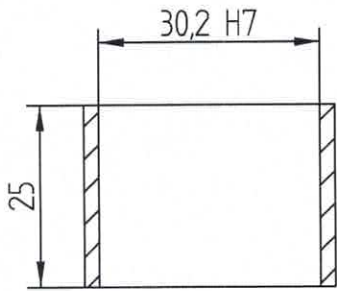
CORTE H-H
