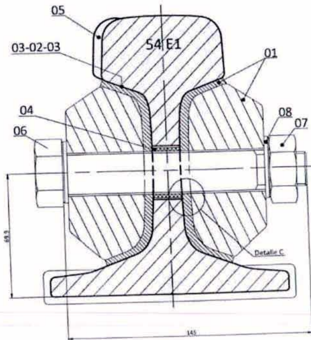
SECCIÓN A-A
