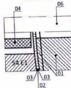
DETALLE C
