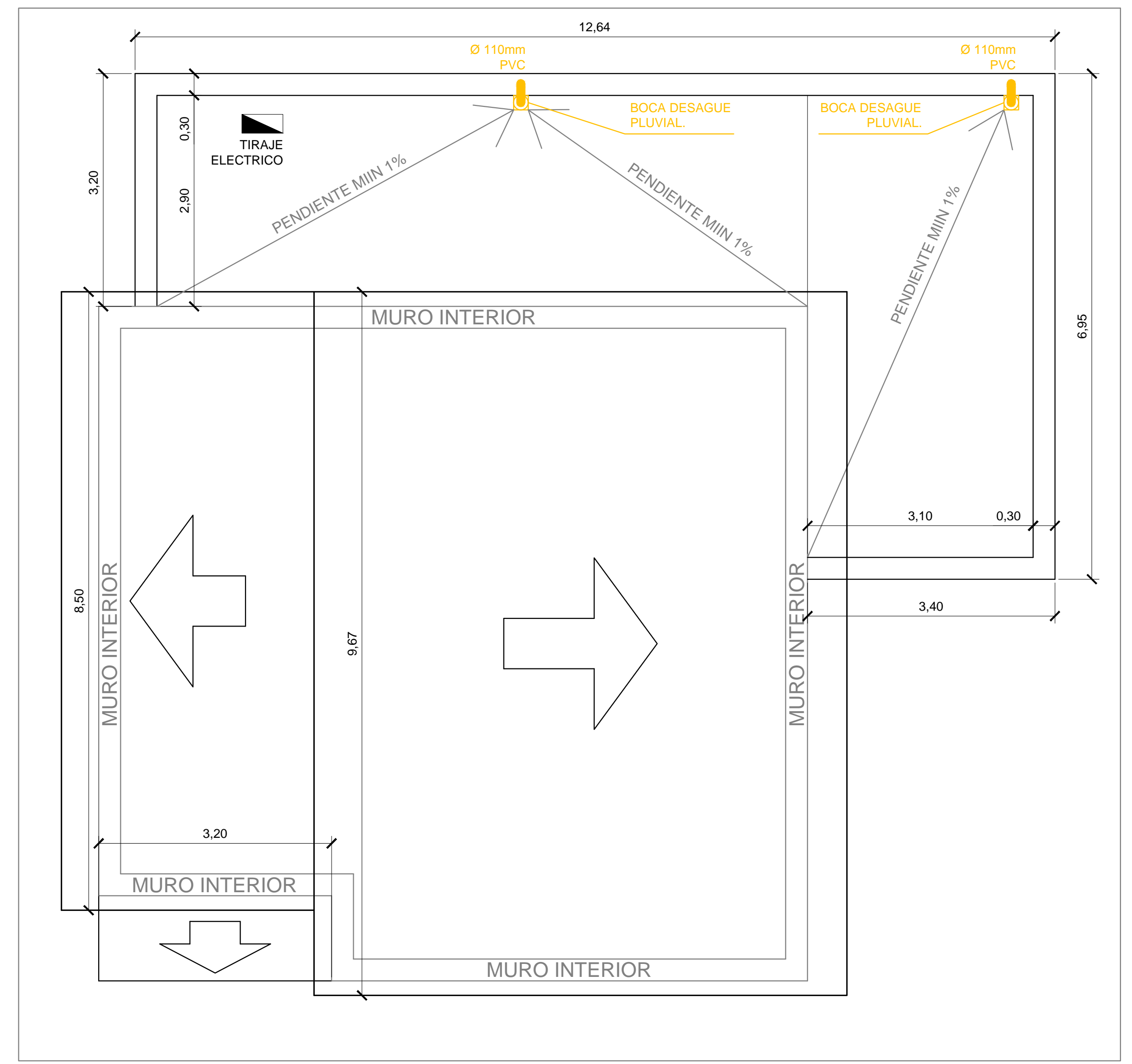
ANTEPROYECTO - INSTALACION SANITARIA Y PLUVIAL PLANTA DE TECHO. ESCALA 1/50
