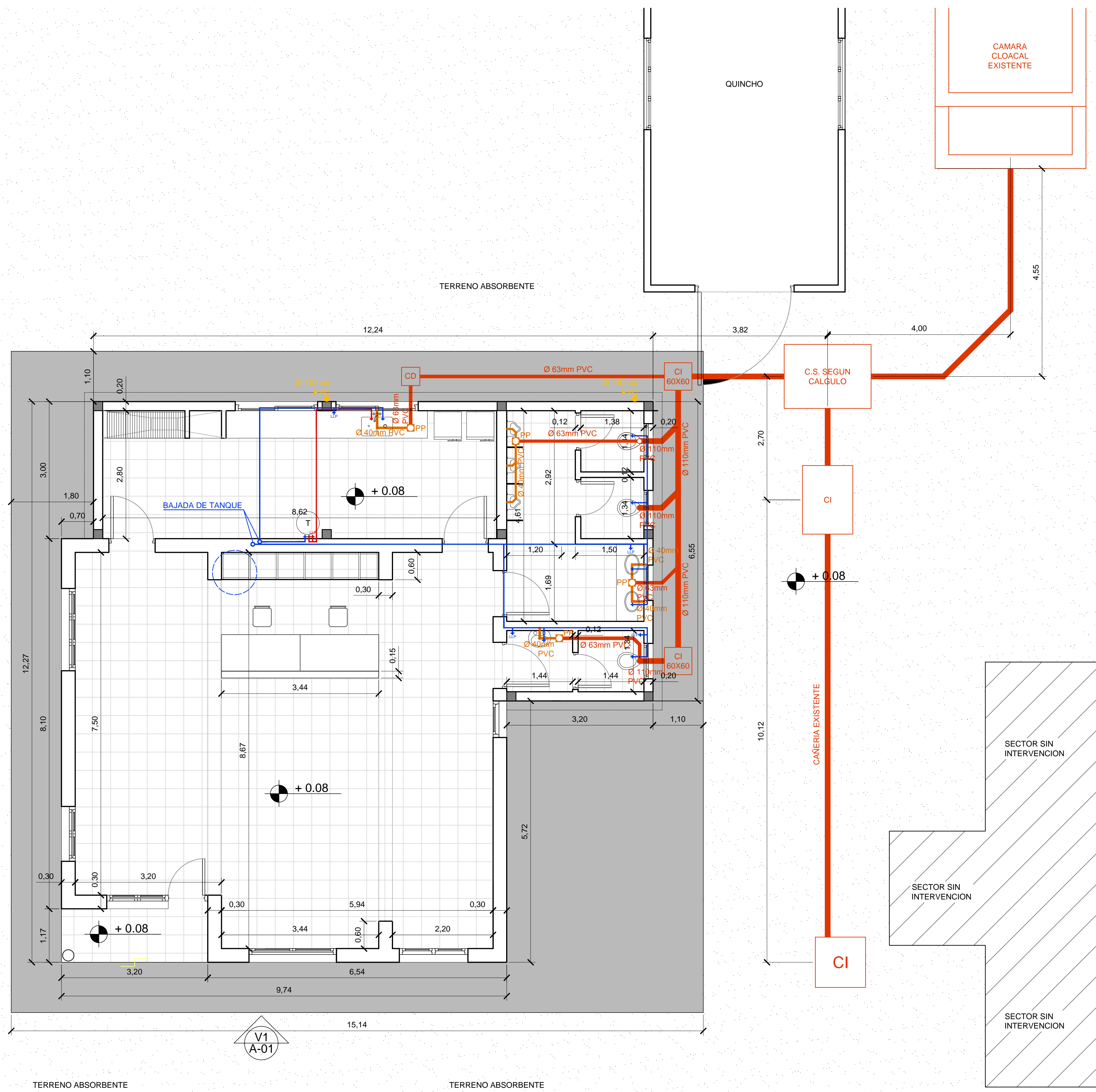
ANTEPROYECTO - INSTALACION SANITARIA Y PLUVIAL PLANTA DE TECHO. ESCALA 1/50
