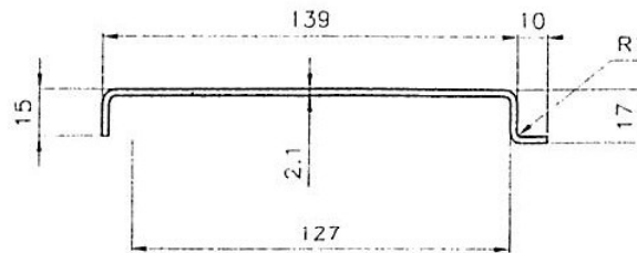
CHAPA BWG N°14 ACERO F24
