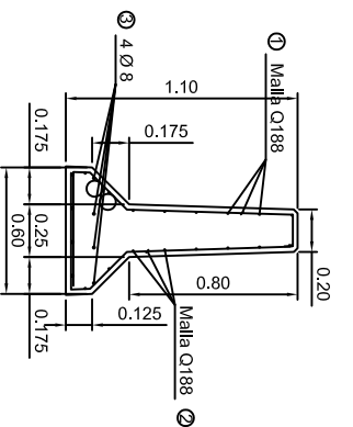
DETALLE ARMADURA ESC.: 1:20
