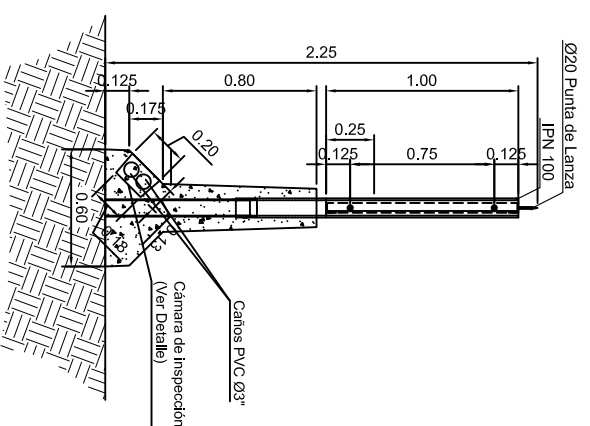
CORTE ESC.: 1:20
