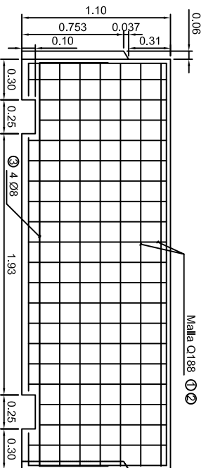
DETALLE ARMADURA ESC.: 1:20
