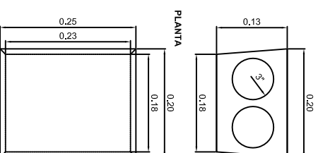
DETALLE CÁMARA DE INSPECCIÓN ESC.: 1:5
