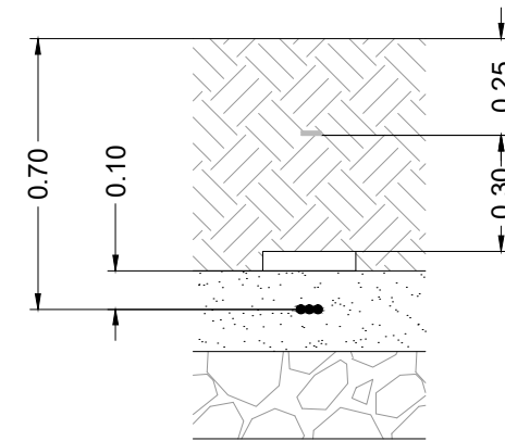
Corte A-A
