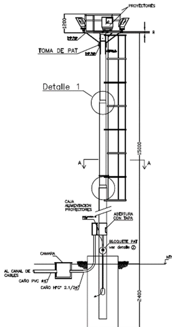
Imagen 10 – Detalle de Torre de iluminación (Ver Anexo X)
