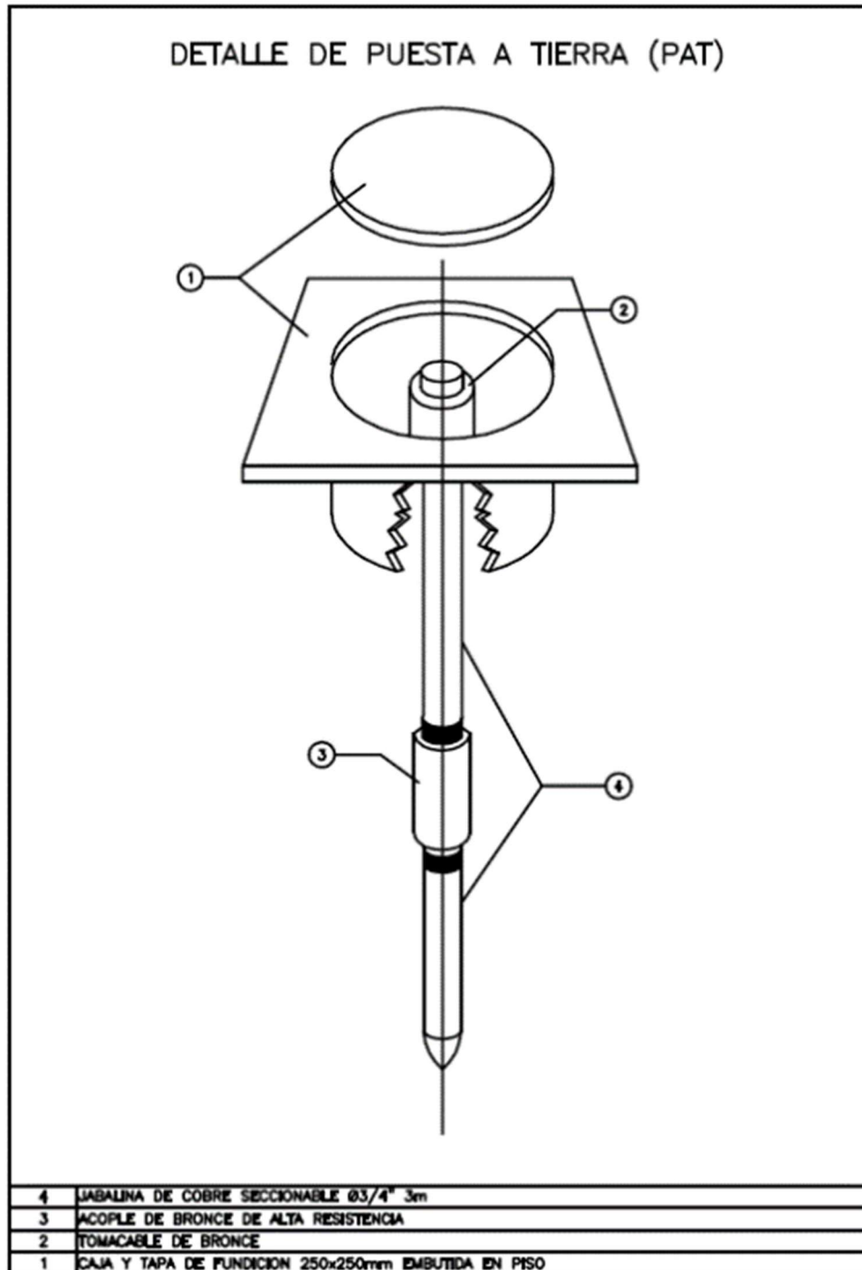
Imagen 11 – Detalle de Puesta a Tierra (PAT)
