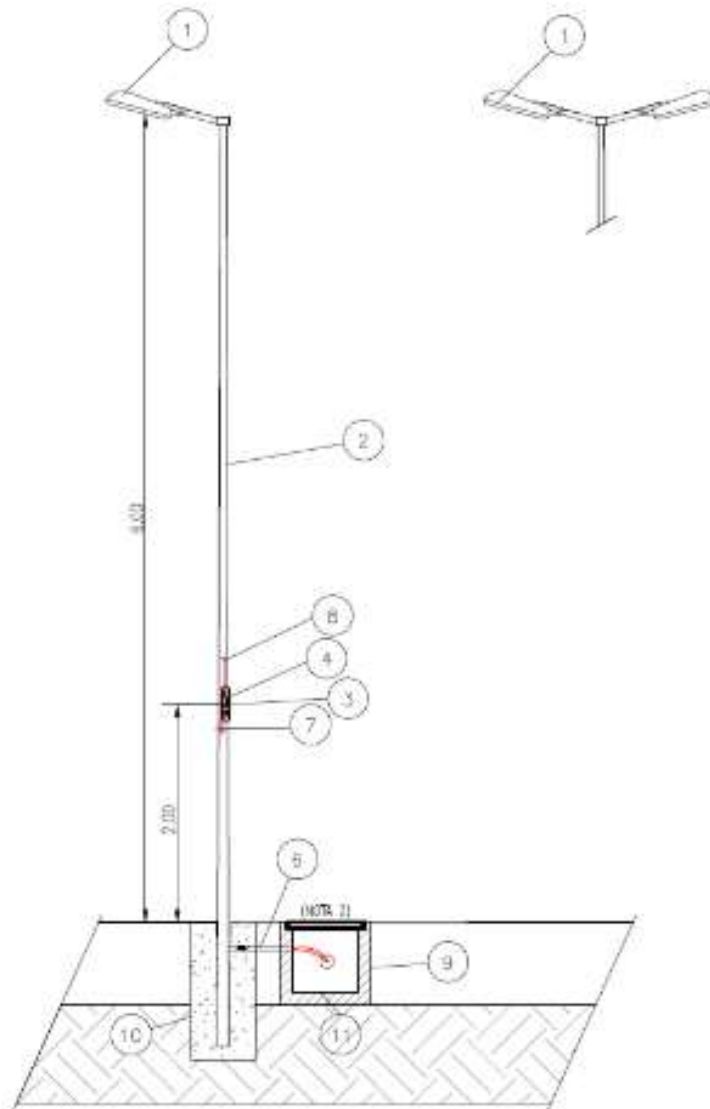
Imagen 9 - Detalle columna de Iluminación (Ver Anexo X)
