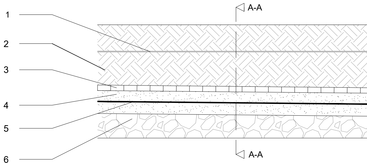
Corte Longitudinal
