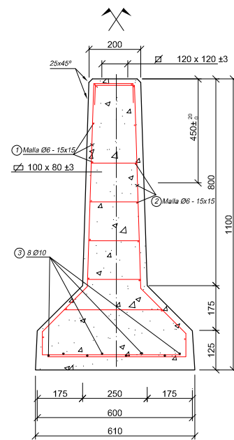
CORTE B - B
