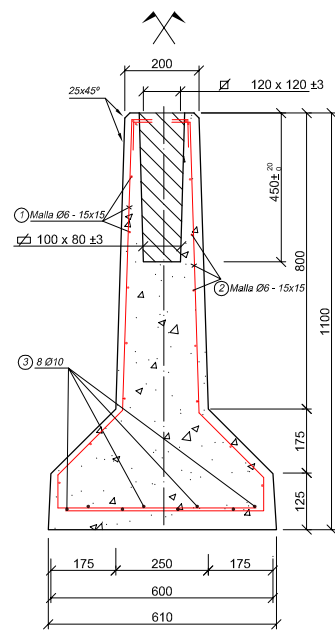
CORTE A-A
