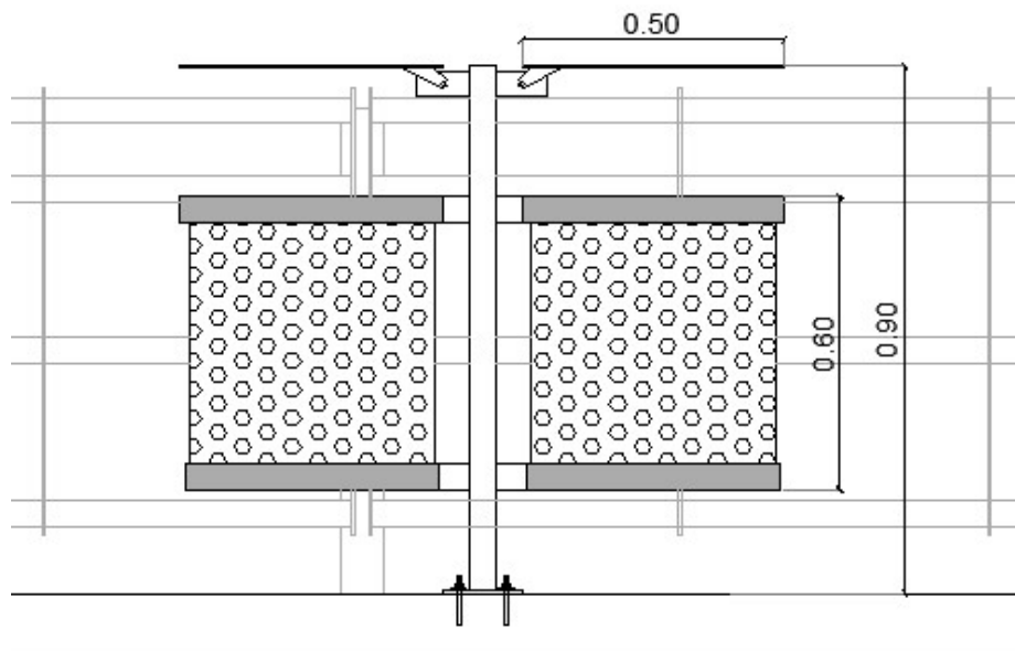
Imagen 18: Detalle de Cesto Papelerero sobre andén
