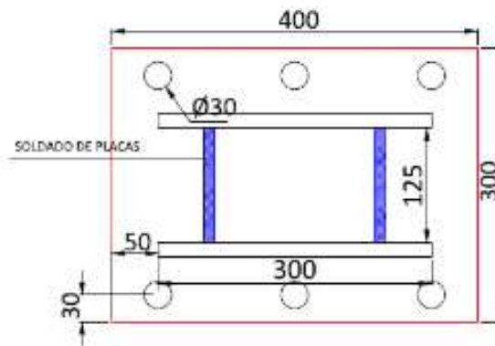
Imagen 15: Detalle placa base
