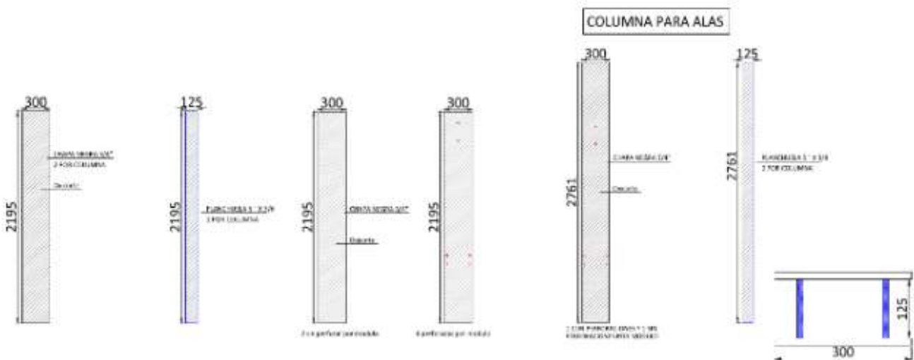
Imagen 14: Detalle columnas por módulo
