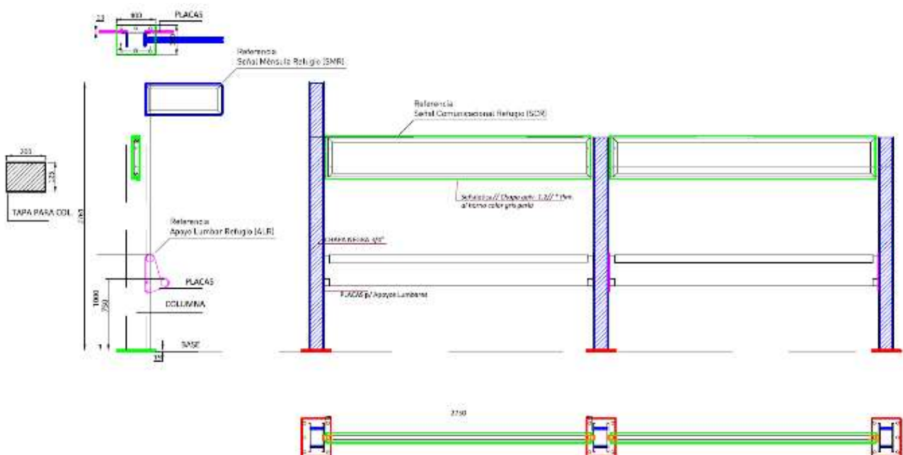
Imagen 13: Esquema Señales Comunicacionales con Apoyo Lumbar
