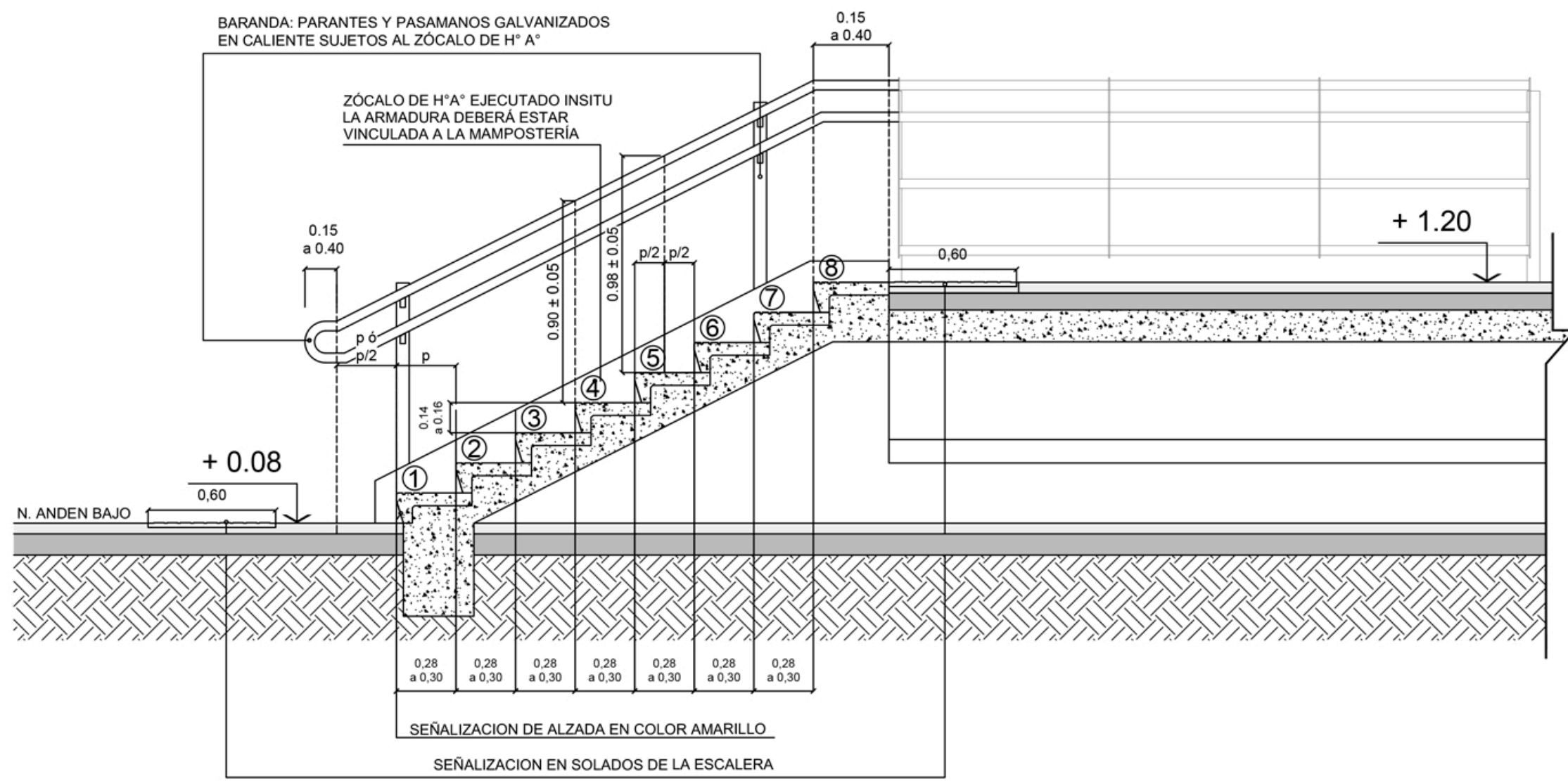
VISTA ACCESO TÍPICO ESC: 1:25
