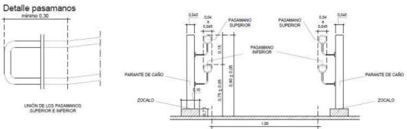
Imagen 8: Detalle de barandas y pasamanos para rampa de acceso
