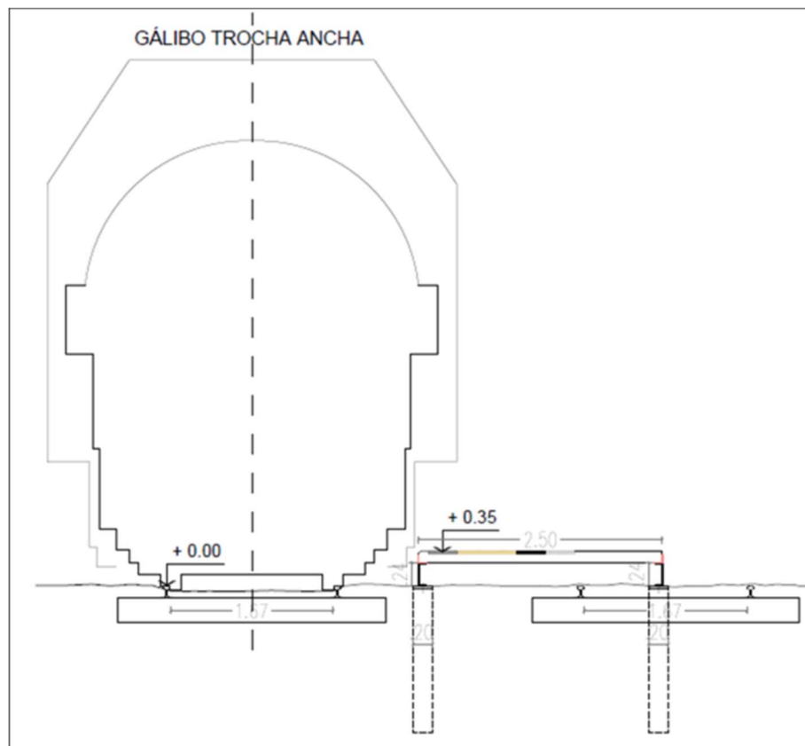
Imagen 6: Corte de Loseta premoldeada a adquirir.
