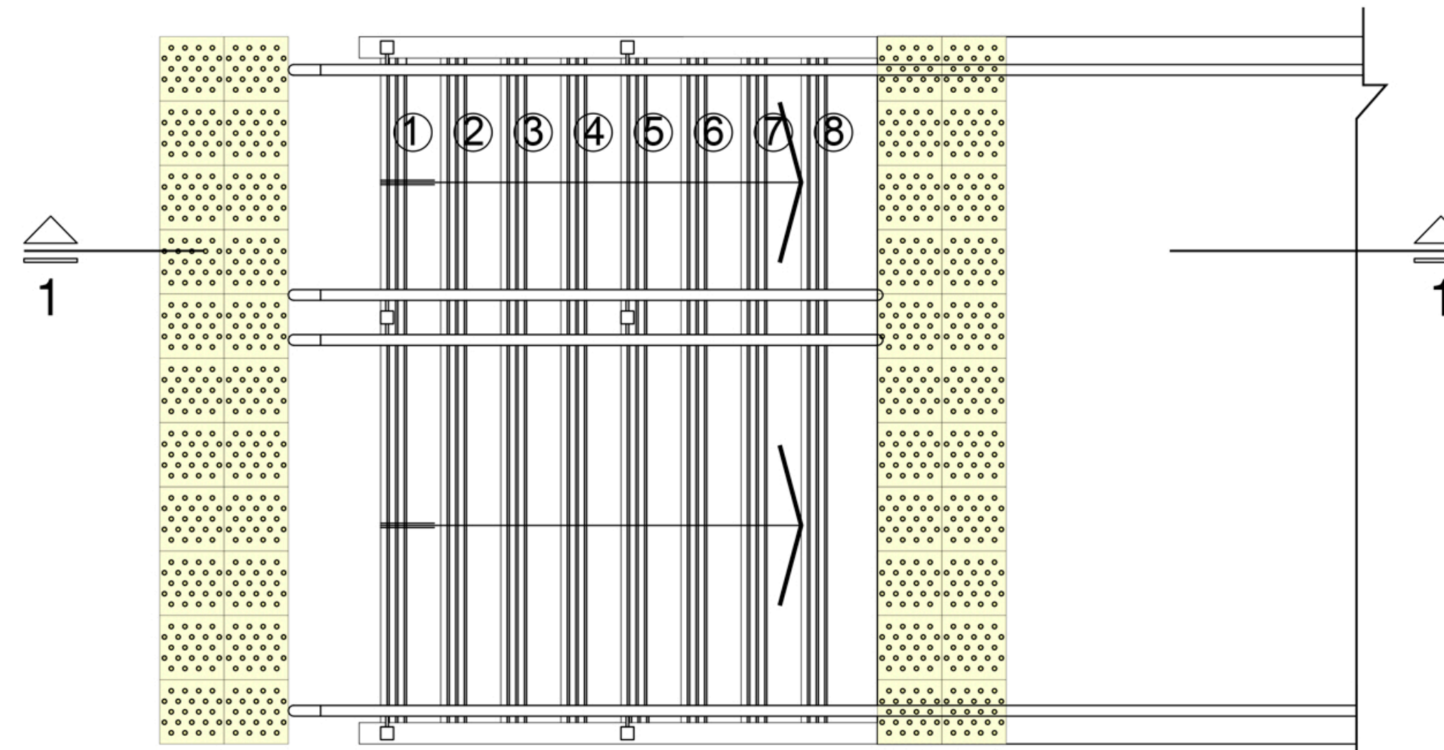
PLANTA ESC: 1:25
