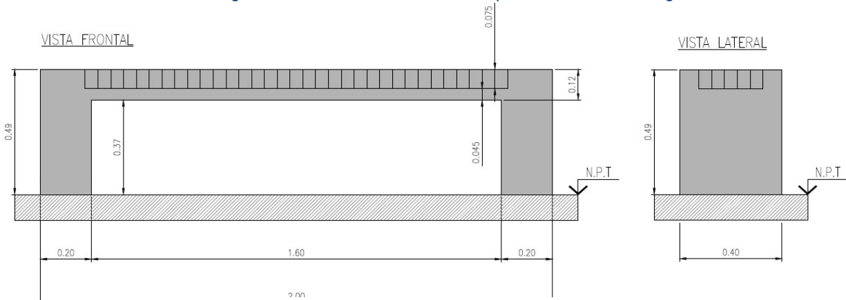
Imagen 21: Detalle Vista frontal y lateral de Banco premoldeado de hormigón
