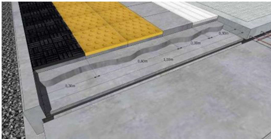
Imagen 7: Detalle de Borde Reglamentario
