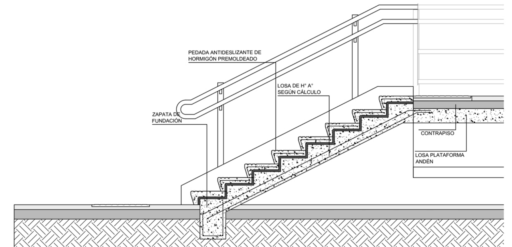
DETALLE ESTRUCTURA SUGERIDO TÍPICO ESC: 1:25
