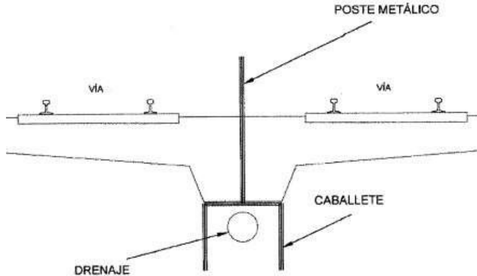
Imagen 24: Detalle Cerco de Entrevía
