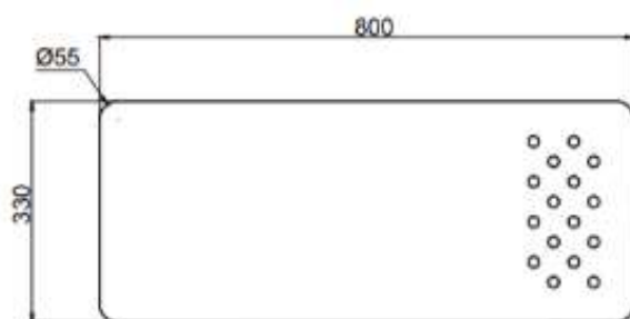
Imagen 11: Esquema Señal Ménsula
