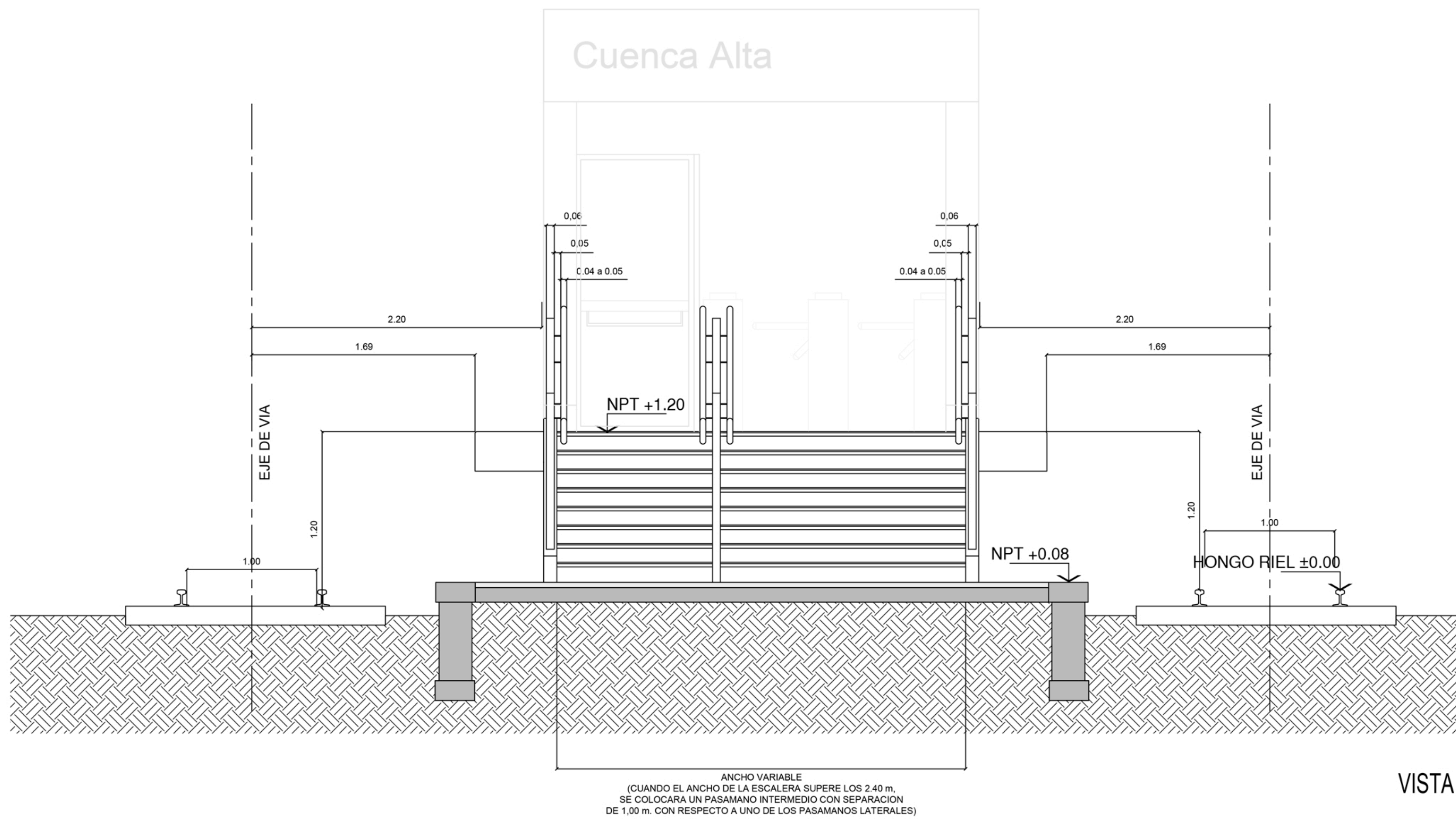
VISTA ACCESO TÍPICO ESC: 1:25
