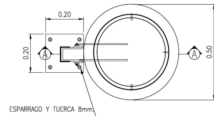
Imagen 17: Detalle en planta de Cesto papelerero
