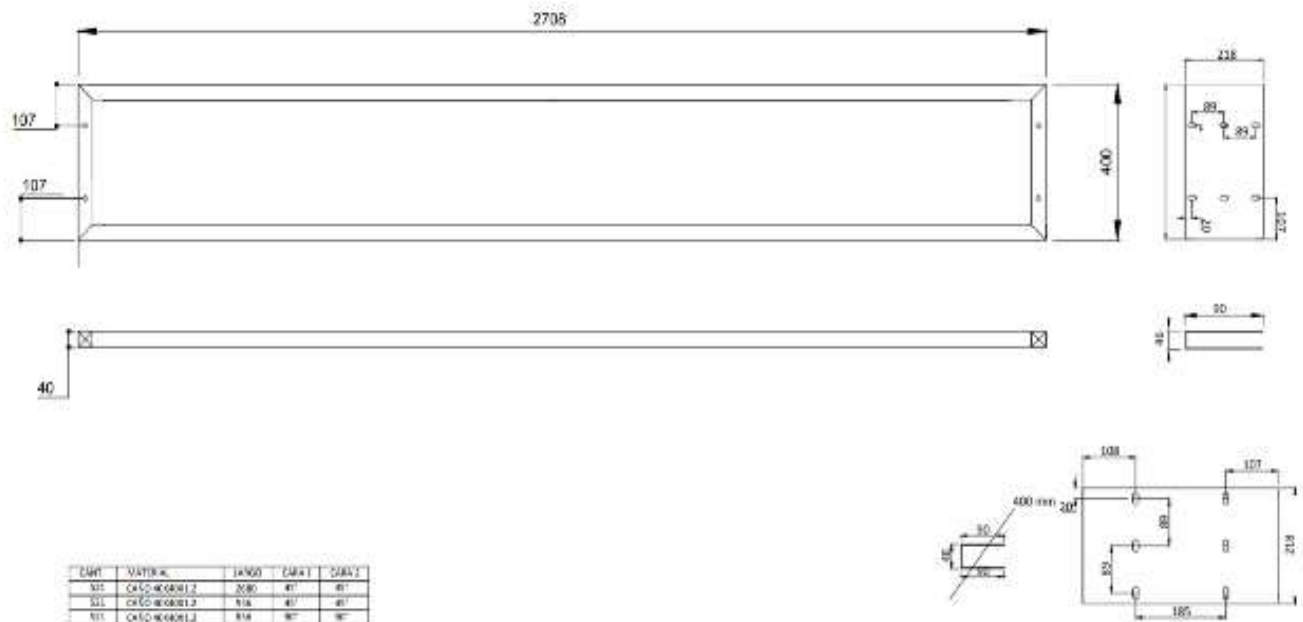
Imagen 10: Esquema bastidor de Señal Comunicacional
