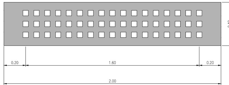
Imagen 20: Detalle en Planta de Banco premoldeado de Hormigón
