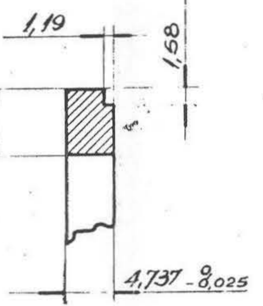
CORTE "LM" ESC: 2:1
