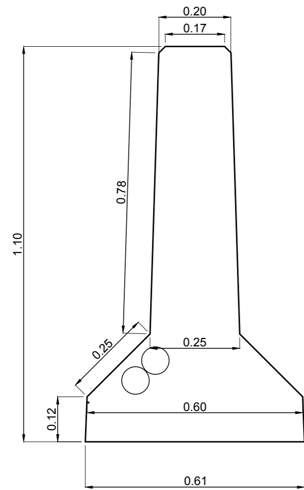
CORTE TRANSVERSAL
