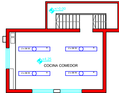
PLANTA 2º PISO
