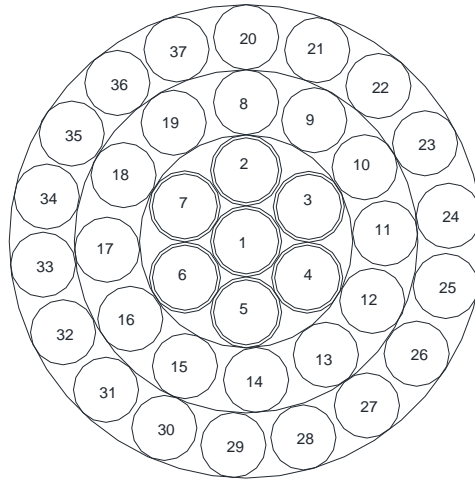
DISTRIBUCIÓN DE PARES CABLE CABLE TRONCAL TELEFONICO
