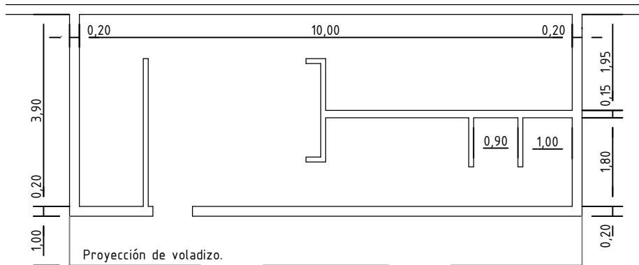
PLANTA: MAMPOSTERIA DE ELEVACIÓN Y LOSA EXISTENTES
