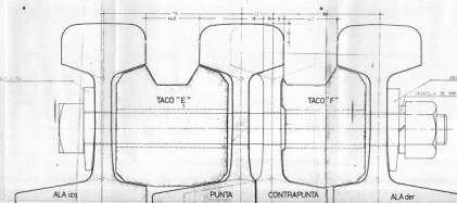
CORTE B-B' (a 1397 mm de Píntal)
