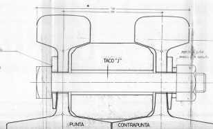
CORTE C-C' (a 1979 mm de Píntal)
