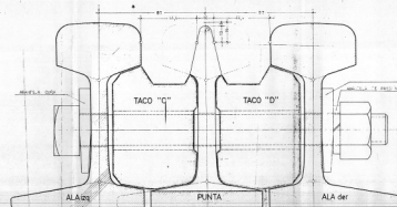
CORTE A-A' (a 150mm de Píntal)
