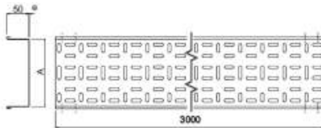
IMAGEN 3.3-2, VISTAS DE BANDEJAS
