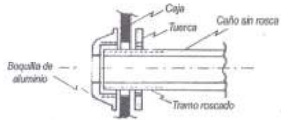
Figura 3.3.2-2. Método de fijación del caño al cubiero o caja.
