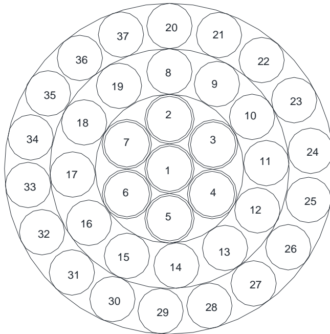
DISTRIBUCIÓN DE PARES CABLE CABLE TRONCAL TELEFONICO
