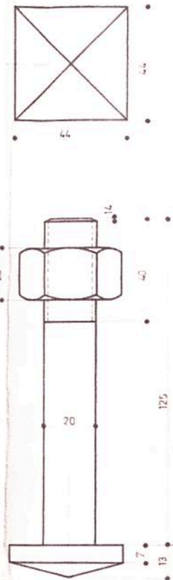
BULON DE CABEZA CUADRADA 20 x 125 (ESC. 1:1)
