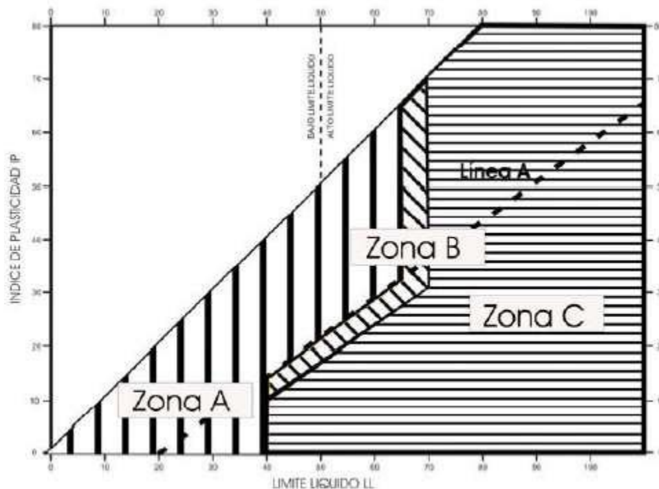
Límites de Atterberg – Suelo apto
