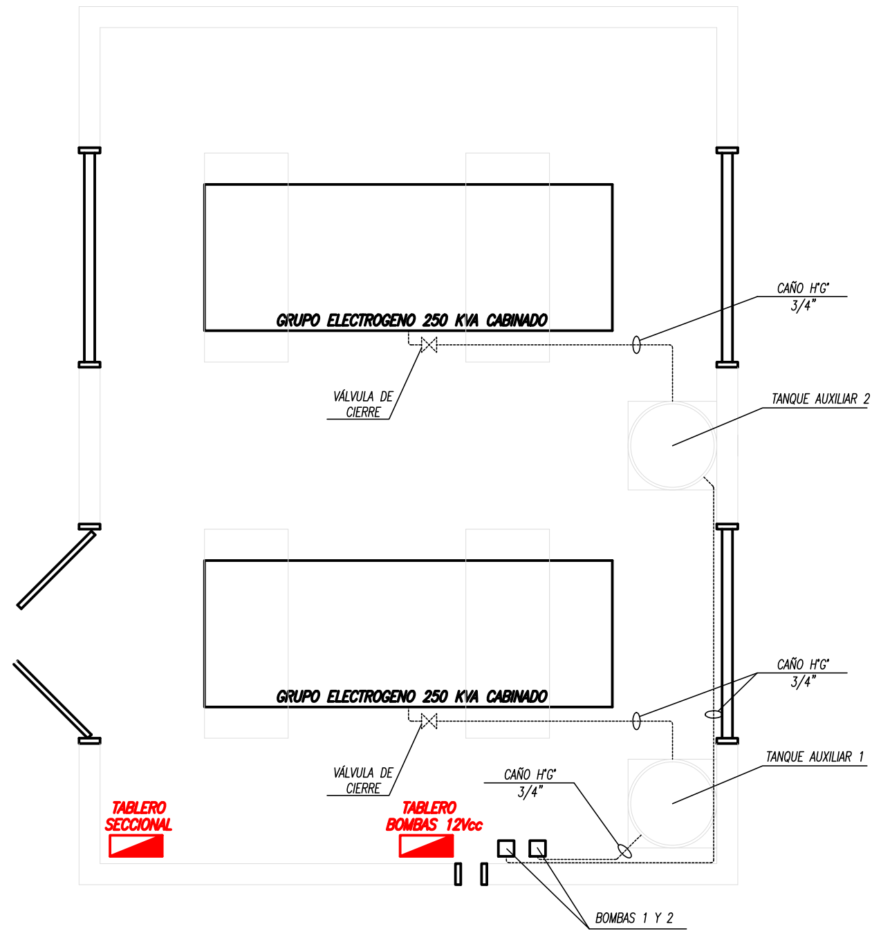
SISTEMA DE CARGA DE COMBUSTIBLE
