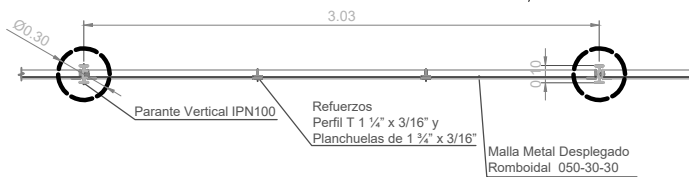
PLANILLA DE MATERIALES POR TRAMO DE 3 M DE REJA DOBLE
