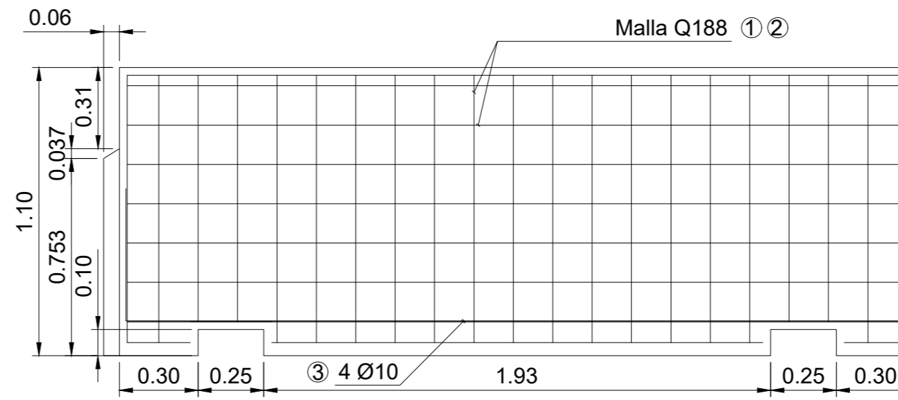
DETALLE ARMADURA ESC.: 1:20
