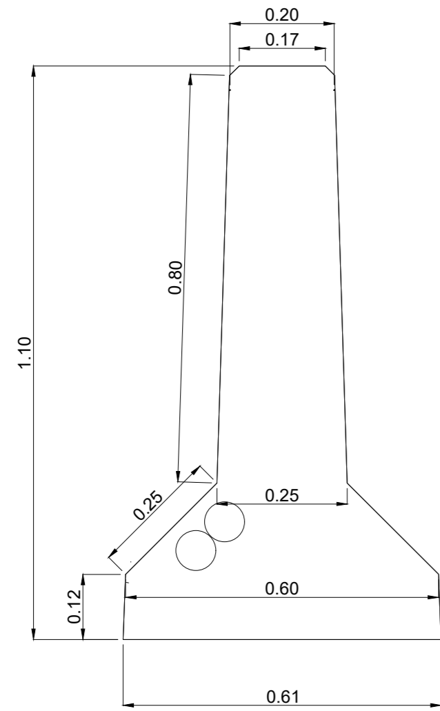
CORTE TRANSVERSAL
