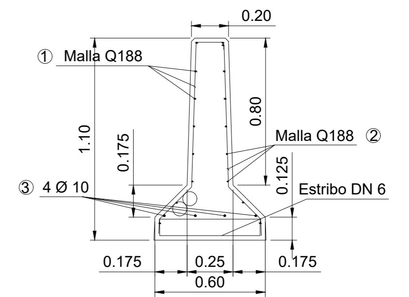
DETALLE ARMADURA ESC.: 1:20
