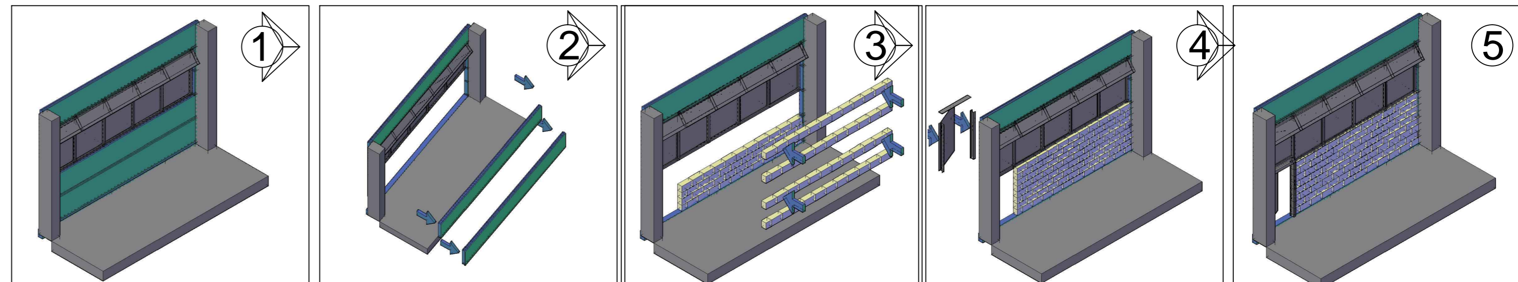
MODULO EXISTENTE RETIRO DE PLACAS PREMOLDEADAS SISTEMA DE CERRAMIENTO BLOQUES HCCA MODIFICACION DE CARPINTERIA PARA INCORPORAR NUEVAS VENTANAS Y PUERTA DE ACCESO MODULO TERMINADO
