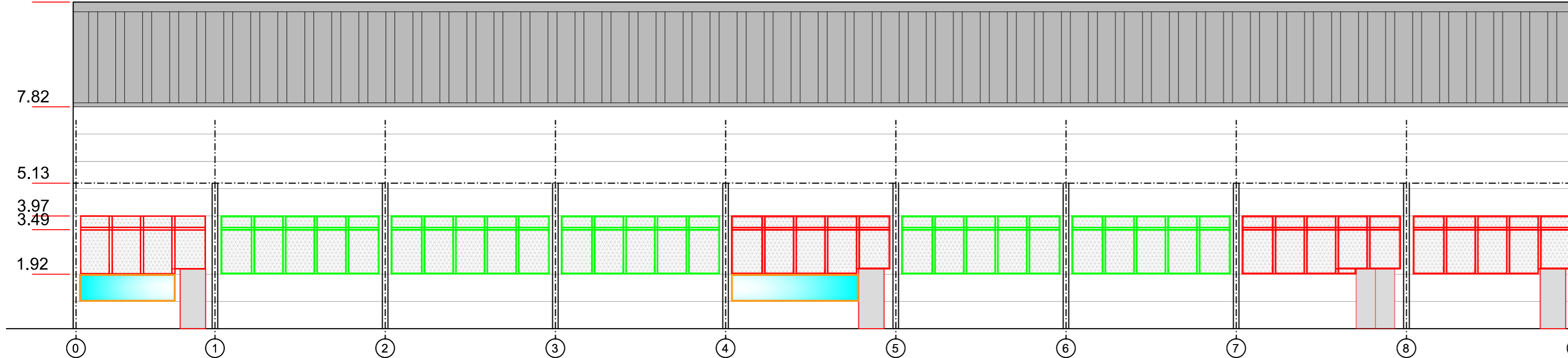
11.51 CORTE A-A /// ANTEPROYECTO
