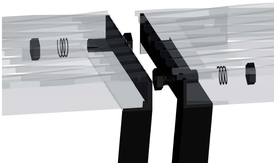
Fijación mecánica individual - vista desde arriba.
