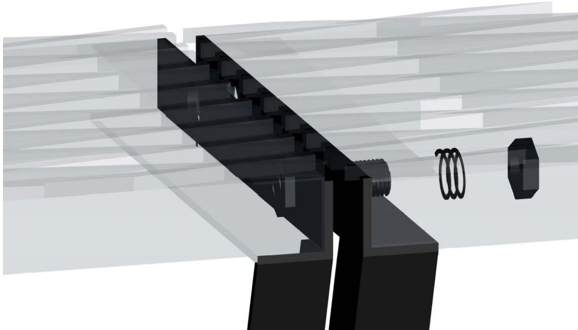
Fijación mecánica continua - vista desde arriba
