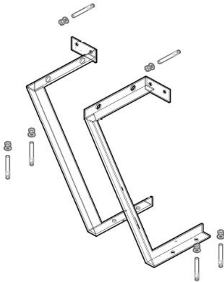
Fijación mecánica superior e inferior.
