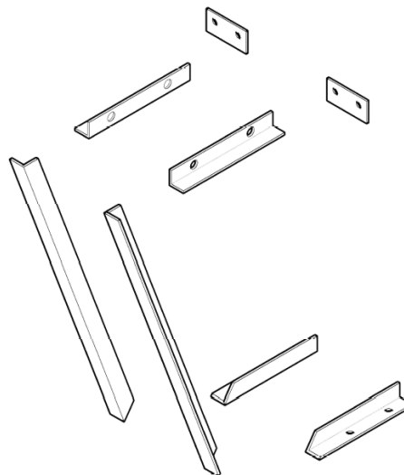
Despiece de estructura soporte
