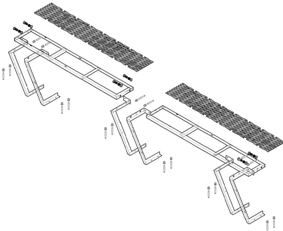
Sistemas de fijaciones mecánicas – fijación continua.
