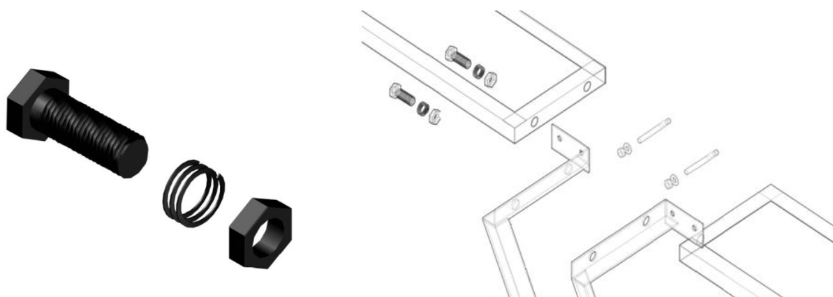
Sistemas de fijaciones mecánicas – fijación continua.
