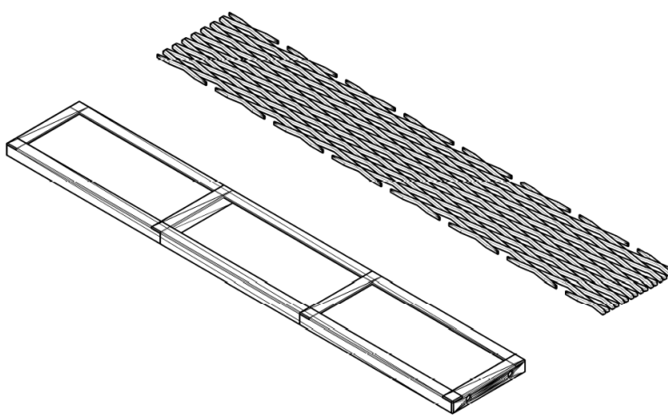
Bastidor con malla tipo shulman (o calidad superior).
