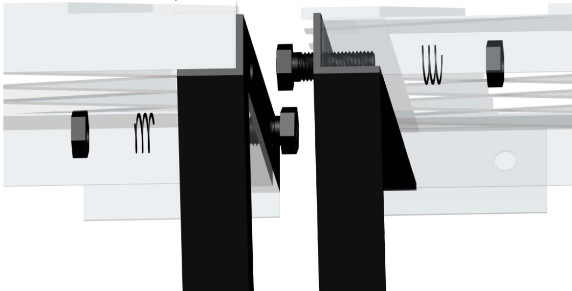
Fijación mecánica individual - vista desde abajo
