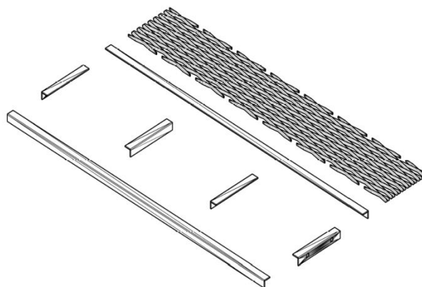
Despiece de plataforma.
