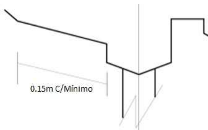
Figura 2. Nueva canaleta a ejecutar
