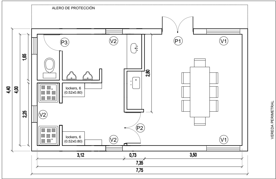
PLANO ANTEPROYECTO
