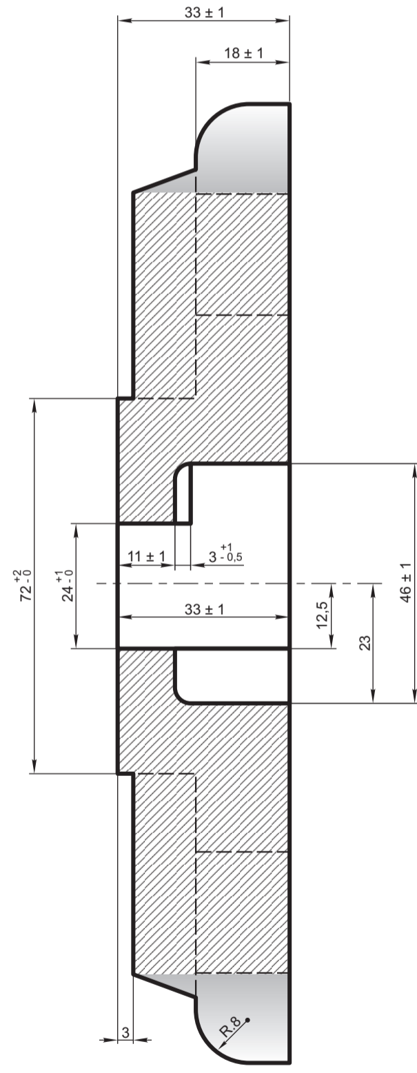
CORTE A-A
