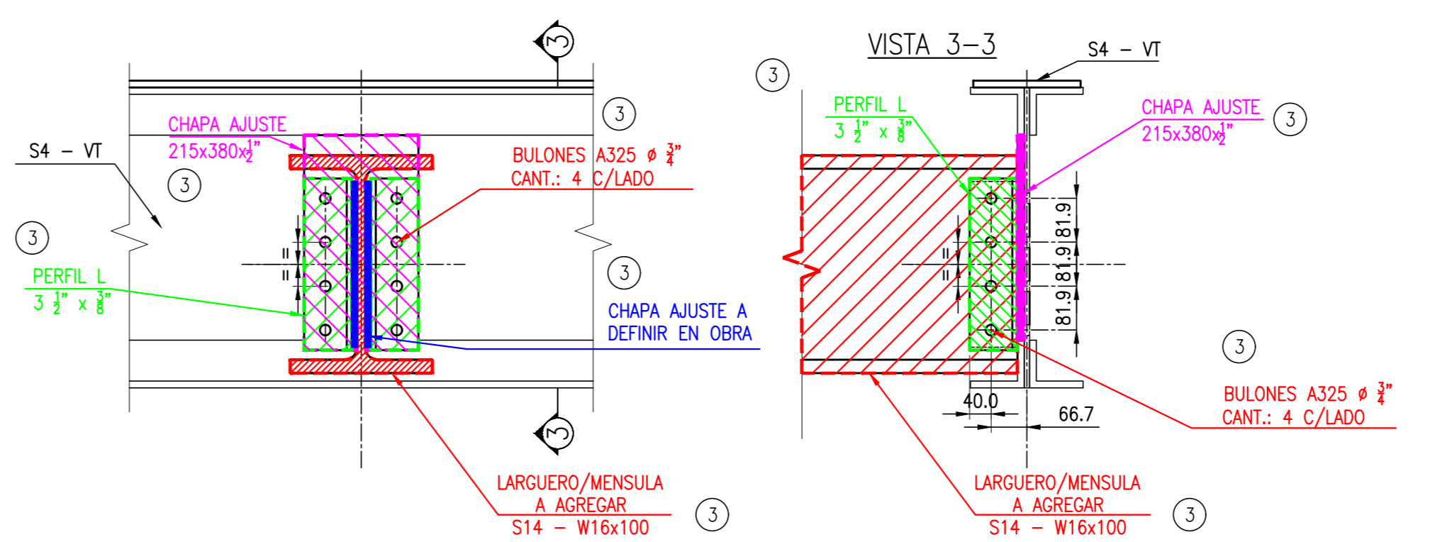
DETALLE 03 ENCUENTRO VIGAS LARGUERO S14 CON VIGA TRANSVERSAL S4 ESC: 1:10
