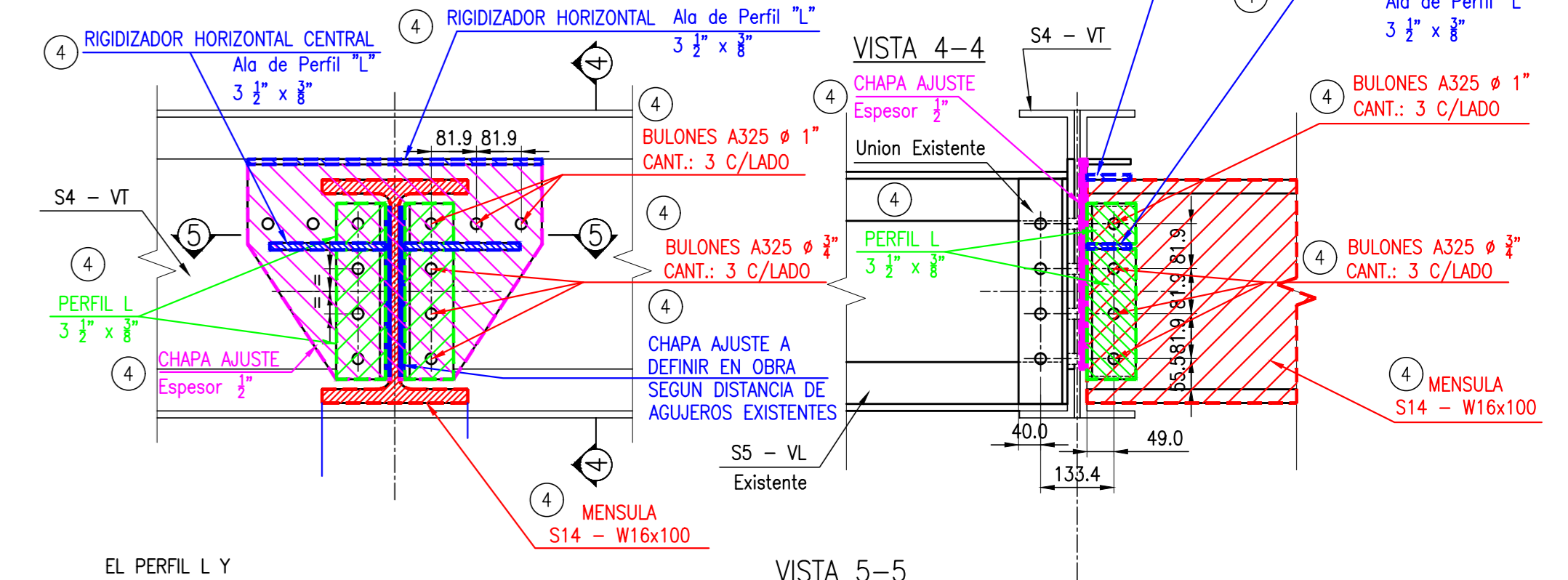
DETALLE 04 ENCUENTRO VIGAS MENSULA S14 Y S5 CON VIGA TRANSVERSAL S4 ESC: 1:10
