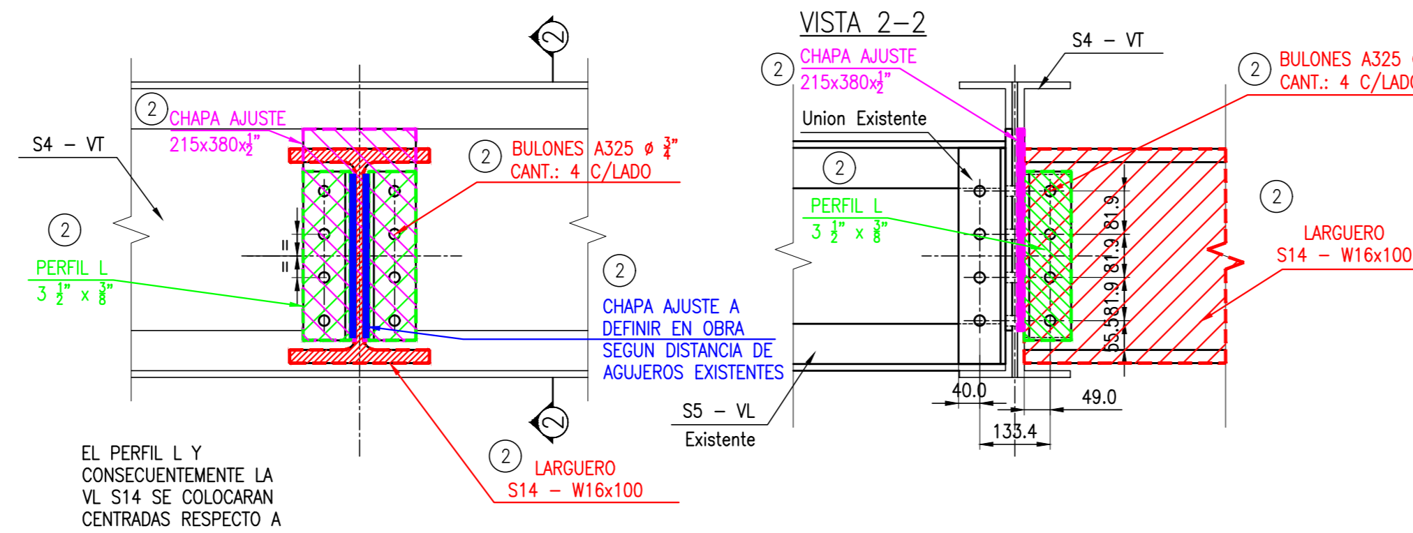
DETALLE 02 ENCUENTRO VIGAS LARGUERO S14 Y S5 CON VIGA TRANSVERSAL S4 ESC: 1:10
