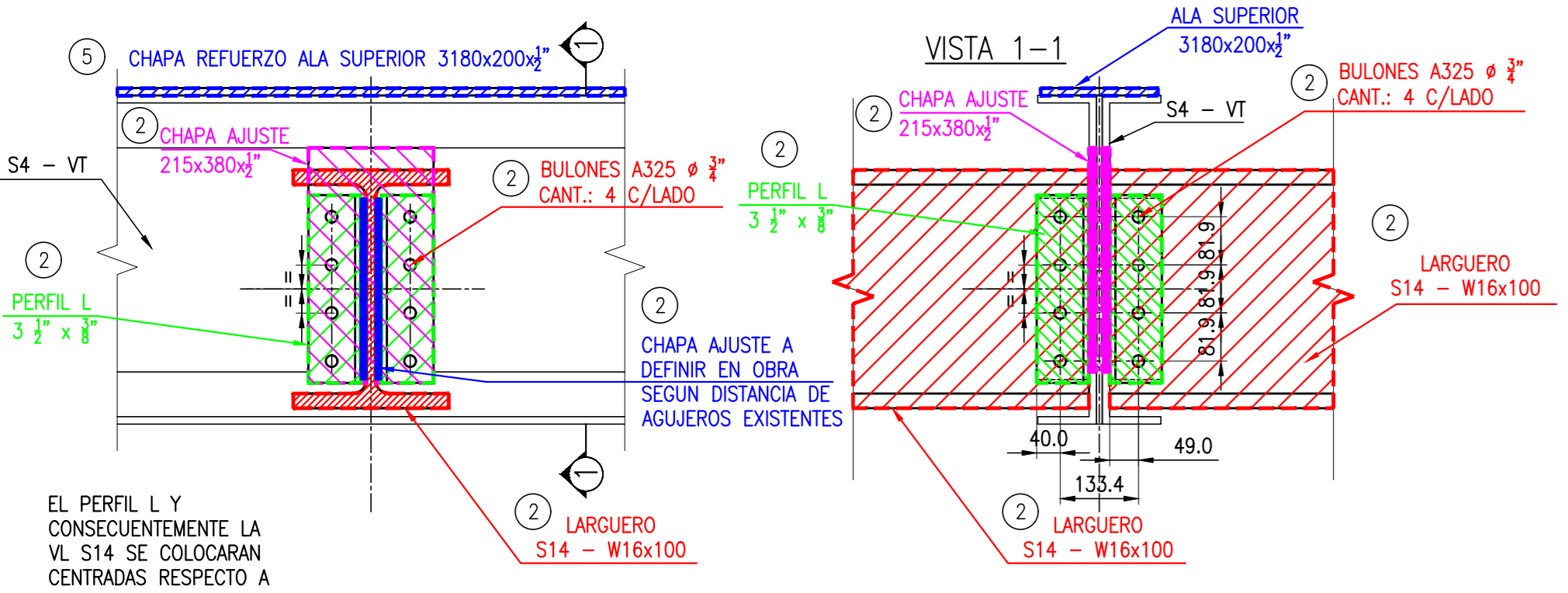
DETALLE 01 ENCUENTRO VIGAS LARGUERO S14 CON VIGA TRANSVERSAL S4 ESC: 1:10
