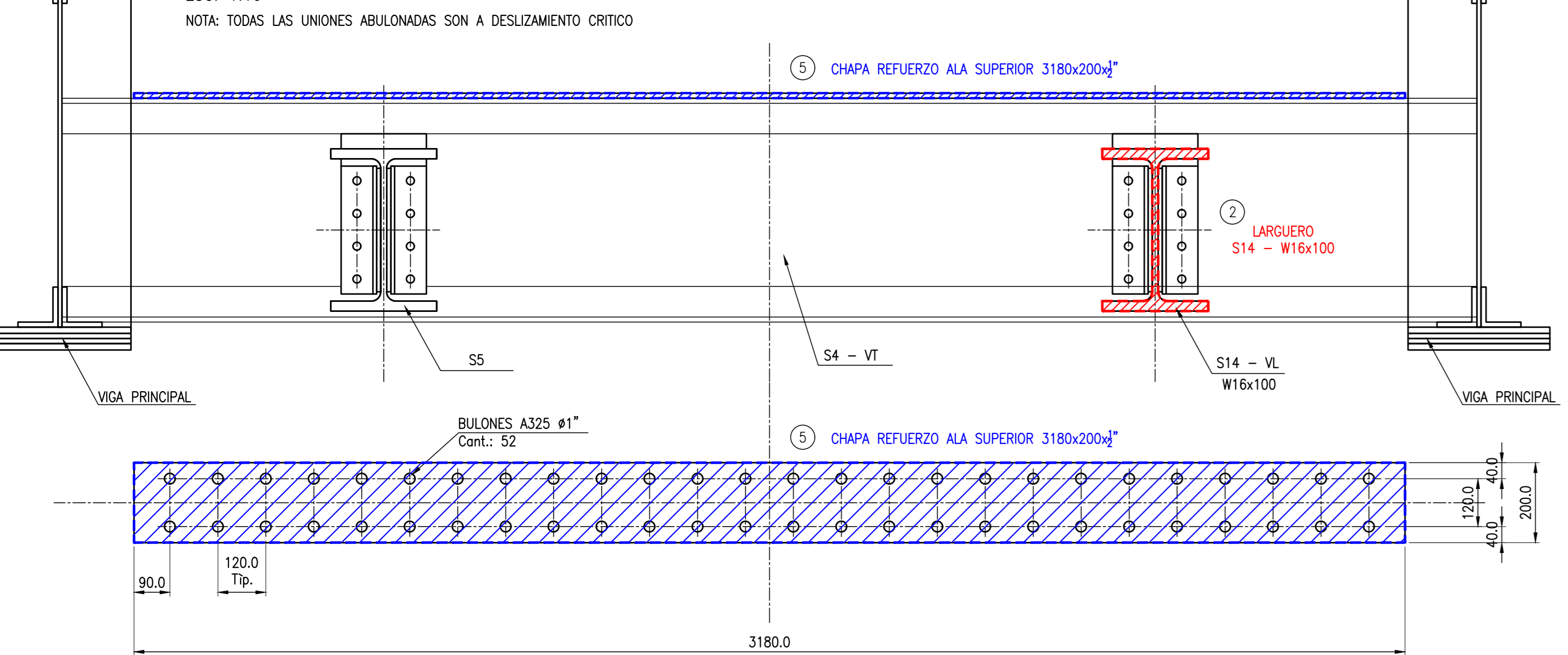
DETALLE 04 ESC: 1:10
