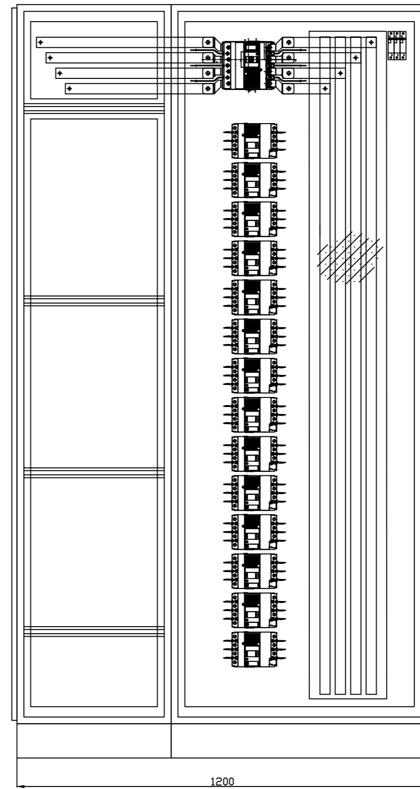
VISTA INTERIOR DISTRIBUCION DE COMPONENTES
