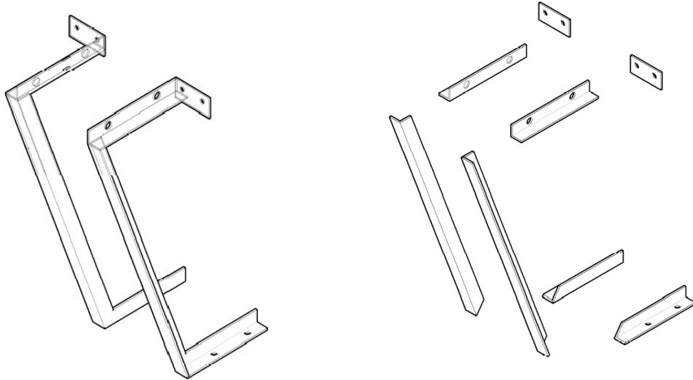
Despiece de estructura soporte
