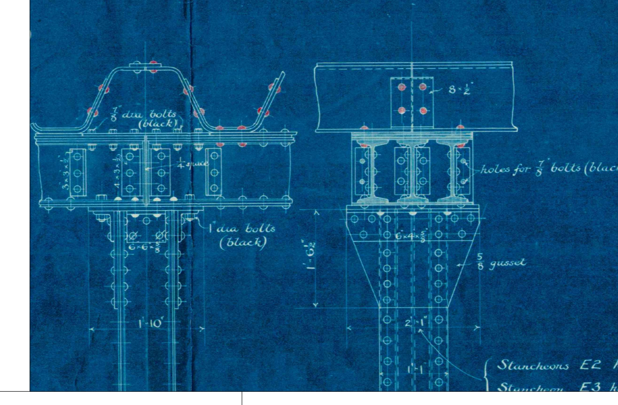
②A DETALLE DE VIGA PRINCIPAL A REEMPLAZAR:
