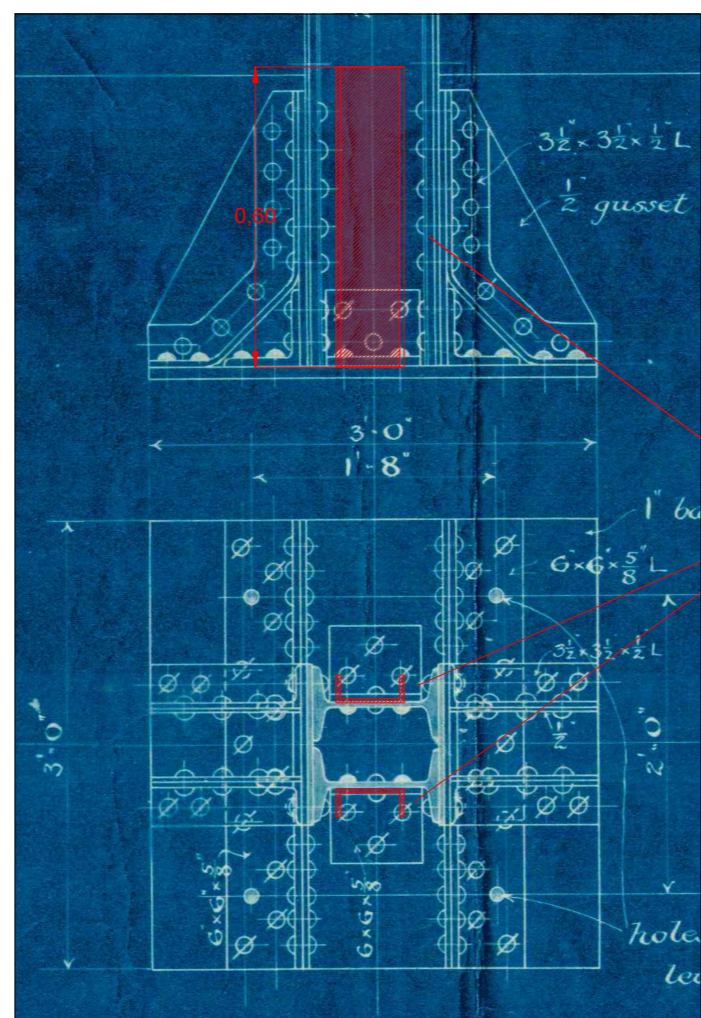
(2B) REPARACION TIPICA DE ARRANQUE DE COLUMNAS
