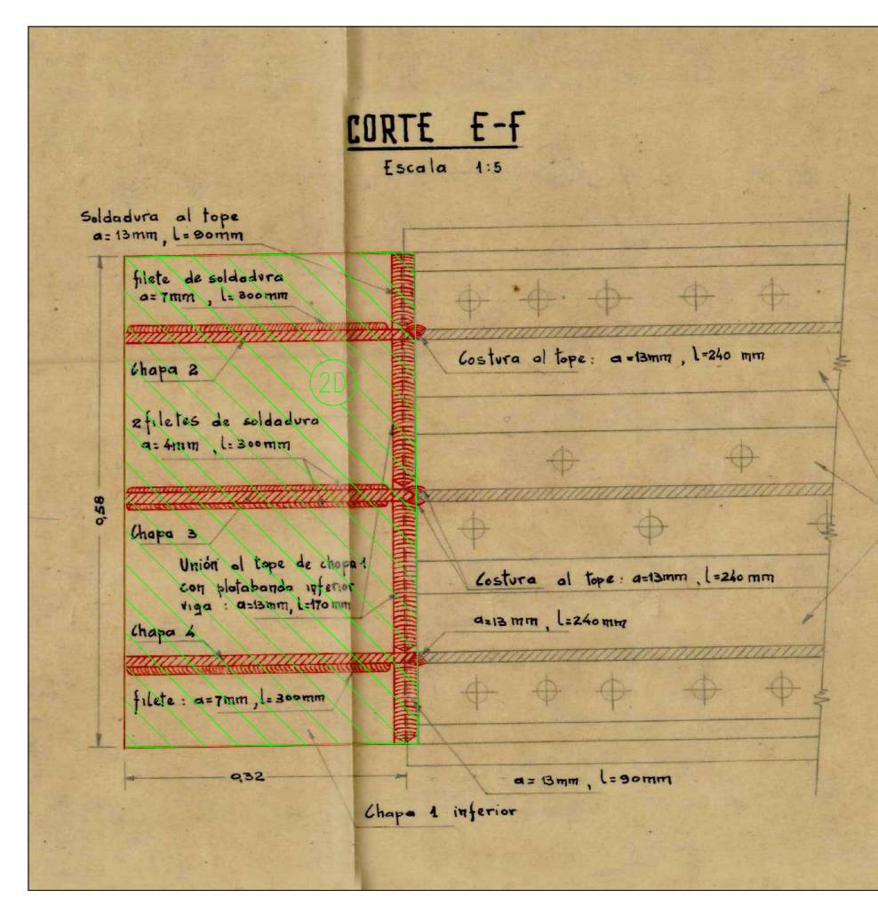
②D DETALLE DE MENSULA
