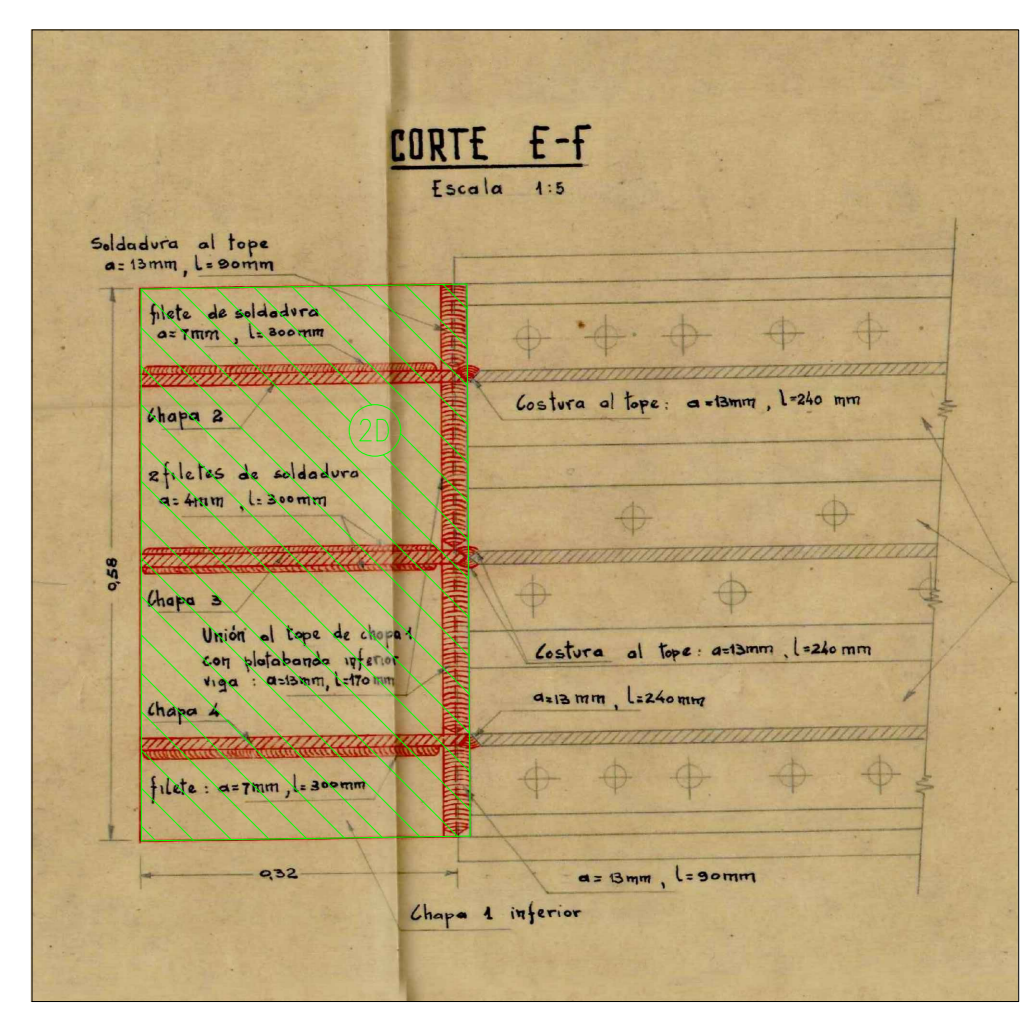
②D DETALLE DE MENSULA
