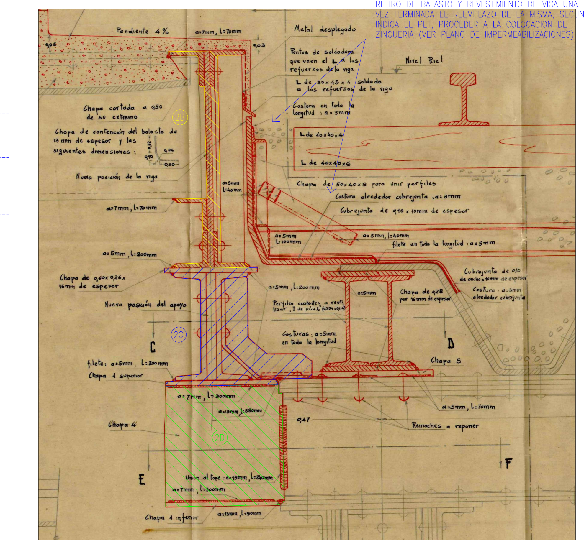
②B ②C ②D DETALLE DE VIGA, PEDESTAL Y MENSULA A REEMPLAZAR:
